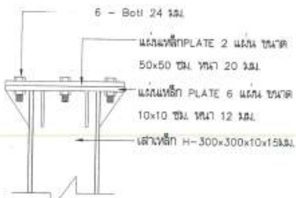
แบบขยาย Plate ยึดโครงสร้างหลังคา มาตราส่วน 1:20
