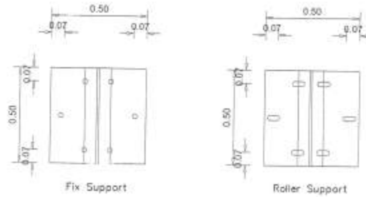
ขยายแผน PLATE หัวเสา มาตราส่วน 1:20
