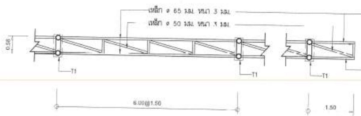
แบบขยาย TRUSS 8 มาตราส่วน 1:75
