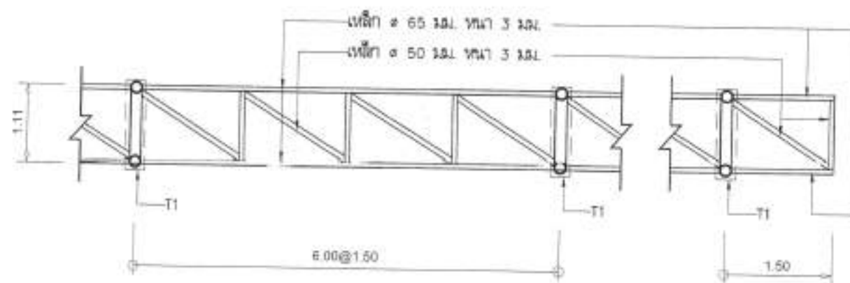
แบบขยาย TRUSS 6 มาตราส่วน 1:75
