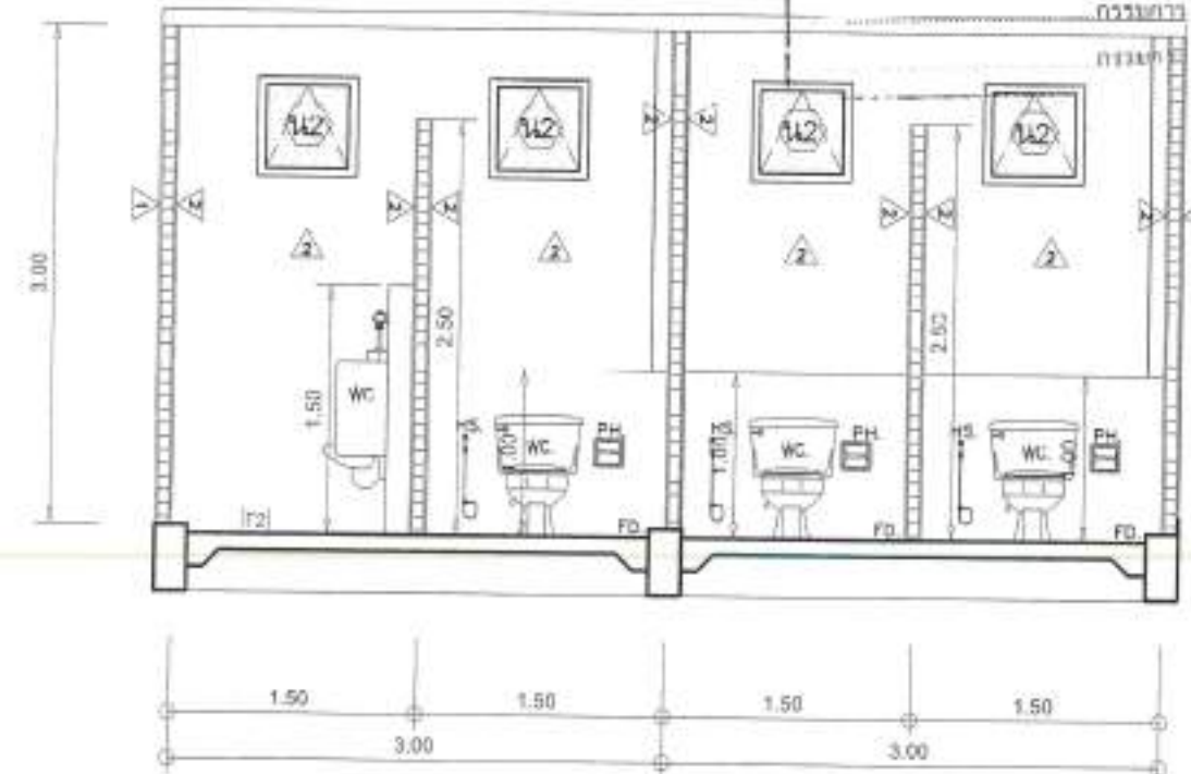
รูปตัด B-B
