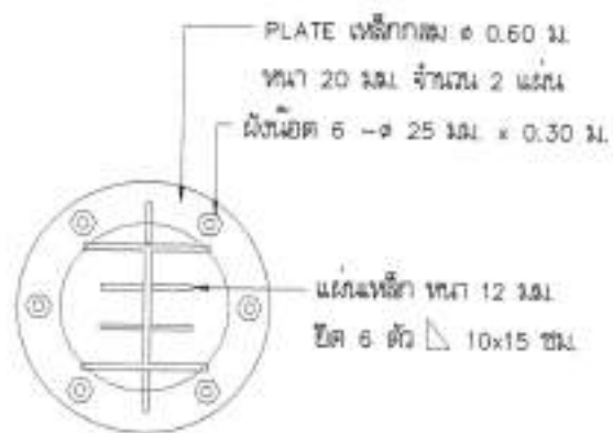
แบบขยาย PLATE เสา คสล. มาตราส่วน 1:20
