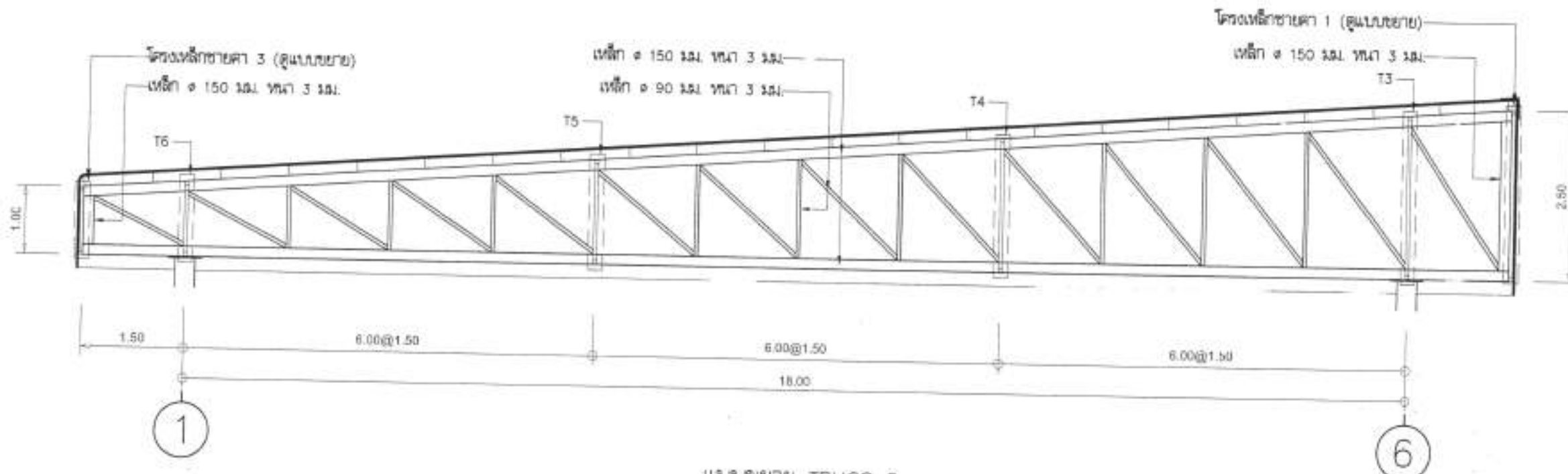
แบบขยาย TRUSS 2 มาตราส่วน 1:75
