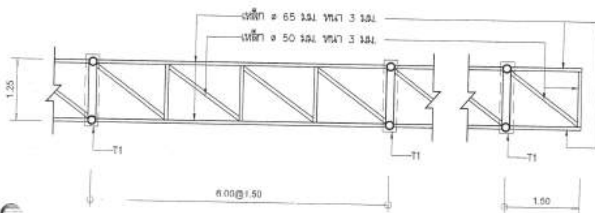
แบบขยาย TRUSS 7 มาตราส่วน 1:75
