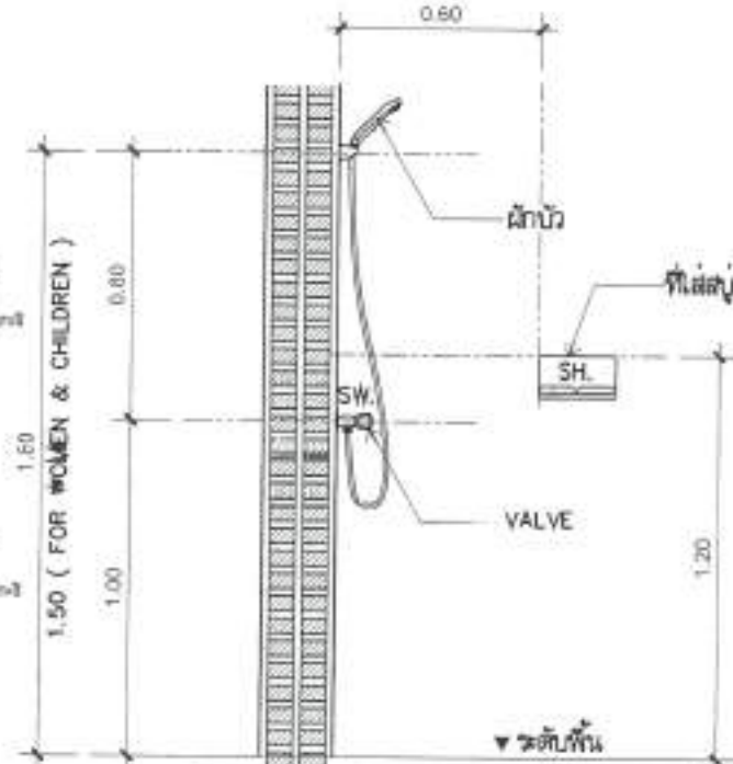
ฝักบัวอาบน้ำ
