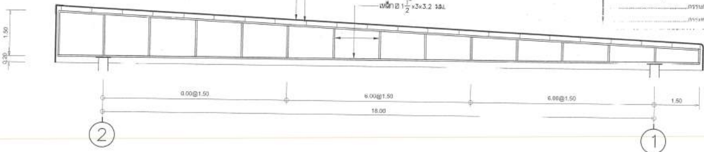
แบบขยายโครงเหล็กปิดข้าง 3 มาตรฐาน 1:75
