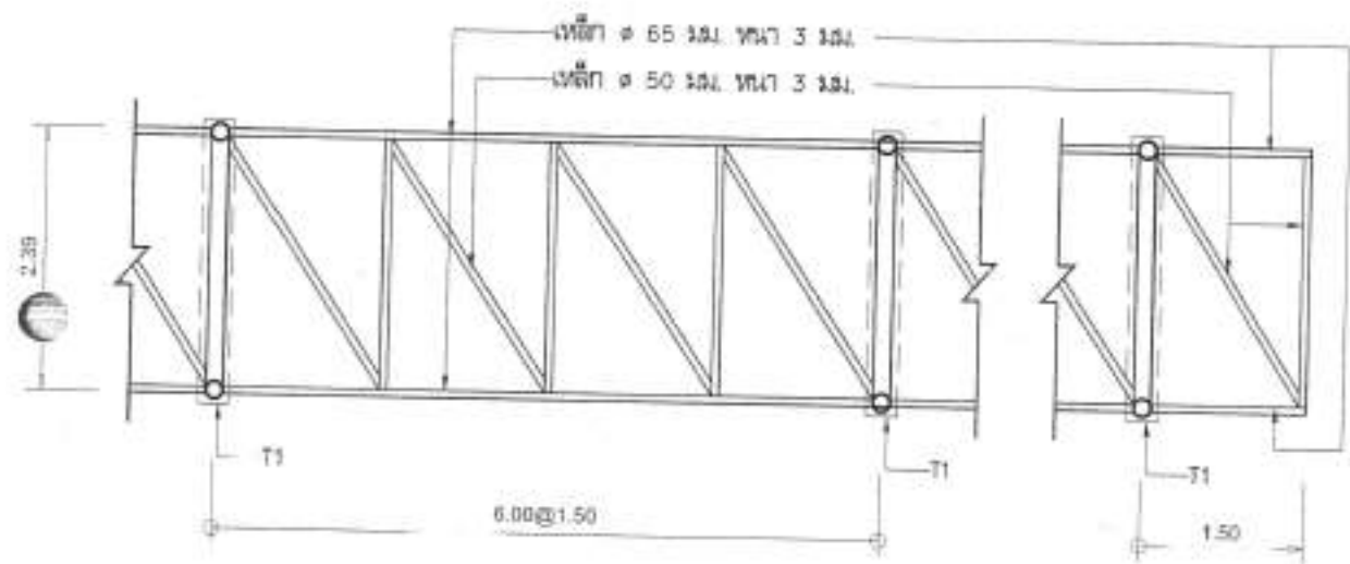
แบบขยาย TRUSS 3 มาตราส่วน 1:75
