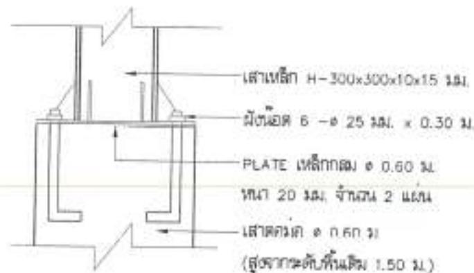
แบบขยาย PLATE ยึดหัวเสา คสล. มาตราส่วน 1:20
