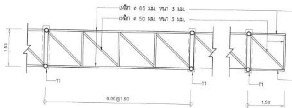
แบบขยาย TRUSS 5 มาตราส่วน 1:75
