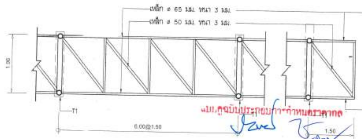
แบบขยาย TRUSS 4 มาตราส่วน
