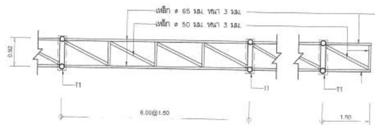
แบบขยาย TRUSS 8 มาตราส่วน 1:75
