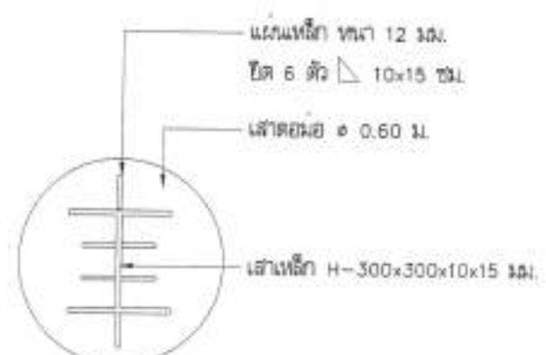
แบบขยายเสาเหล็ก H มาตราส่วน 1:20
