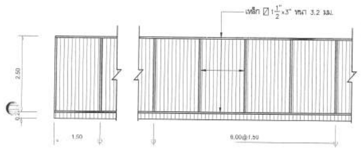
แบบขยายโครงเหล็กชายคา 1 มาตราส่วน 1:75
