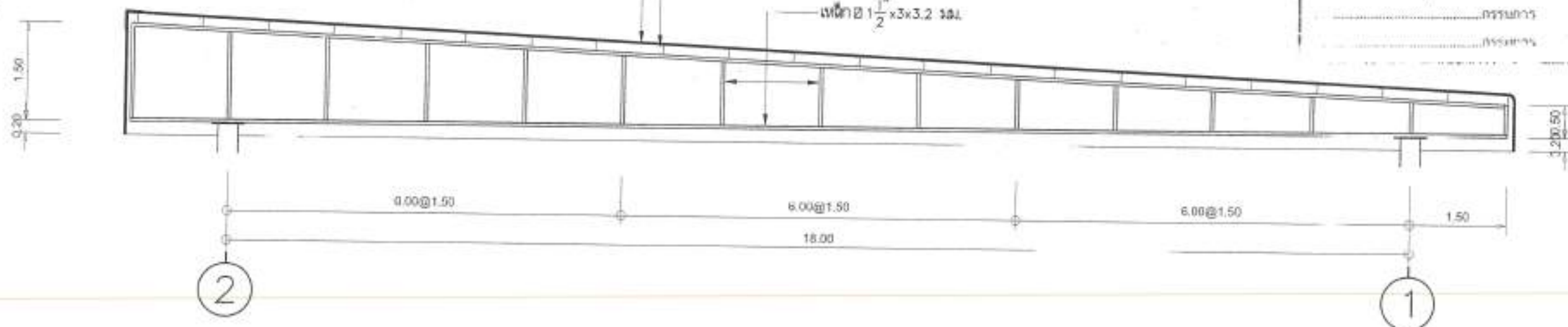
แบบขยายโครงเหล็กปิดข้าง 3 มาตราส่วน 1:75
