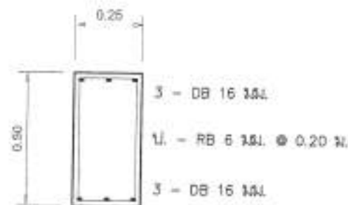
GB1 คานคอดำเนิน
