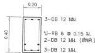
GB2 คานช่วงกลางคาน
