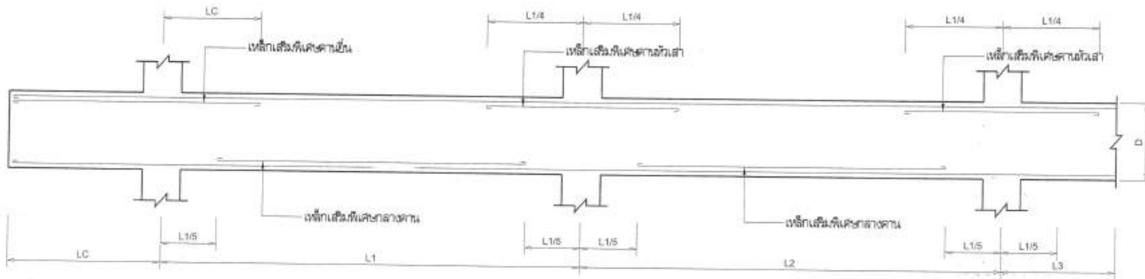
TYPICAL BEAM DSTAILS (แบบขยายมาตรฐานการเสริมเหล็กคาน)
