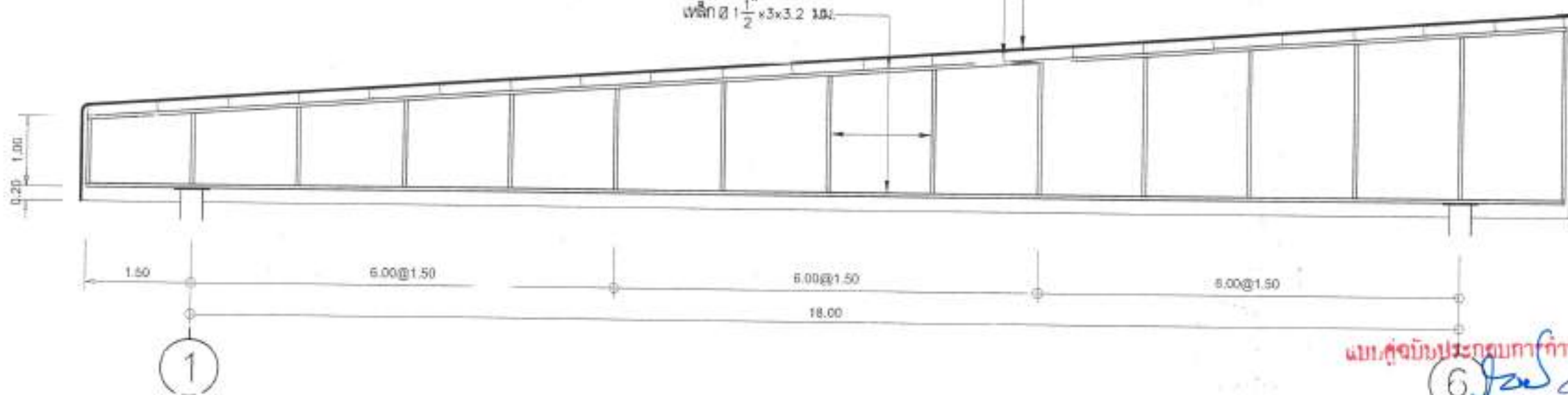
แบบขยายโครงเหล็กปิดข้าง 2 มาตราส่วน 1:75
