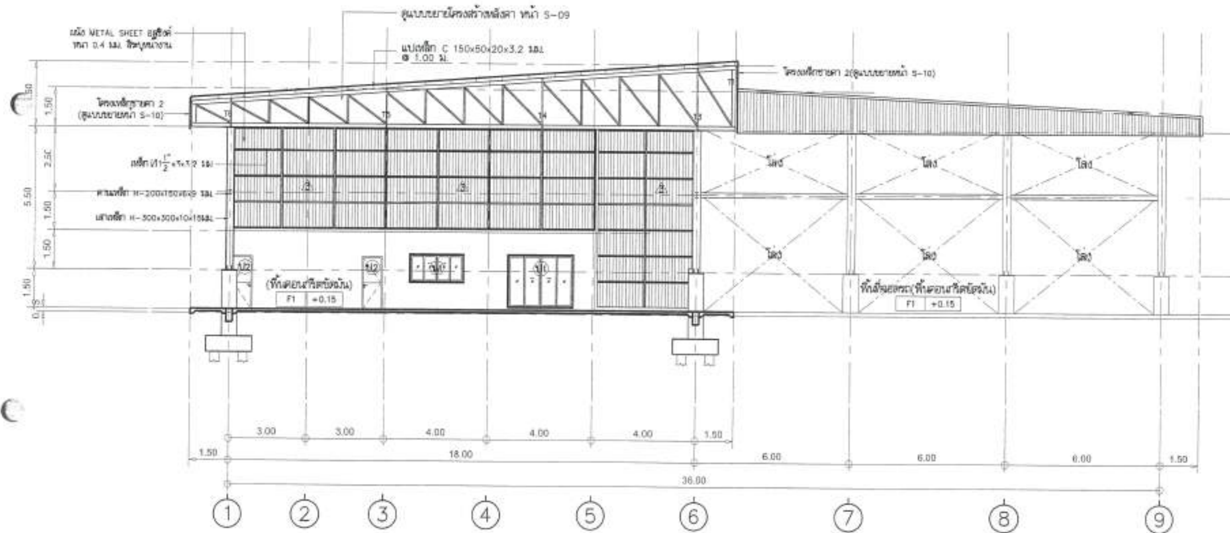
รูปตัด B มาตราส่วน 1:150
