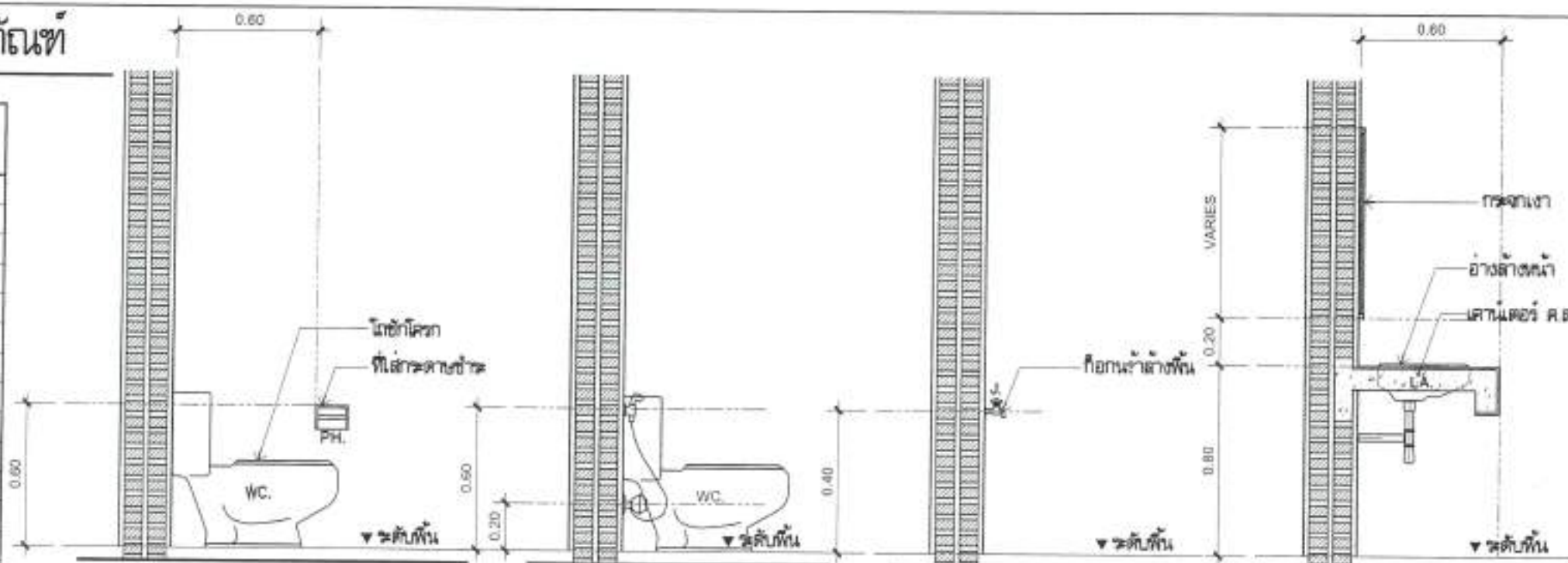
แบบสุขภัณฑ์ประกอบสำเร็จกำหนดราคาติดตั้ง อ่างล้างหน้าชนิดฝังเคาน์เตอร์
