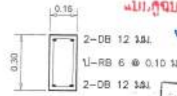
GB3 คานคอดำเนิน
