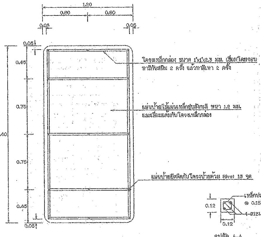
รูปตัด A-A
