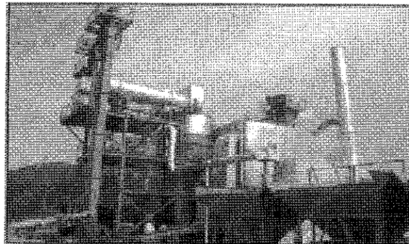
รูปที่ 5 Central Plant แบบ Batch Plant สำหรับผลิต Hot Mix Recycling โดยเฉพาะ
