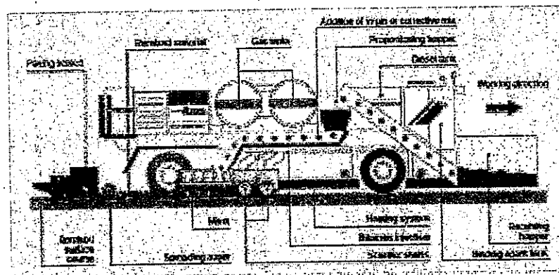
รูปที่ 10 แสดงระบบการทำงานของเครื่อง Re-mixer แบบเปียก (จาก Wirtgen GmbH)
