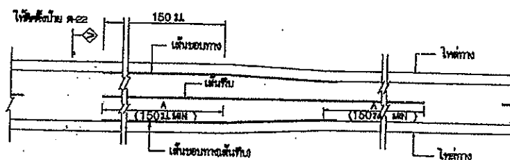
การเว้นระยะจราจร กรณีความกว้างของช่องจราจรลดลง
