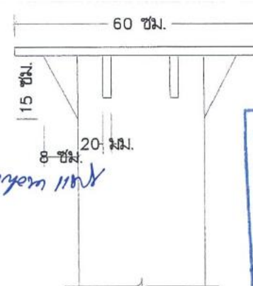
แปลนขยายเพลาหัวเสา
