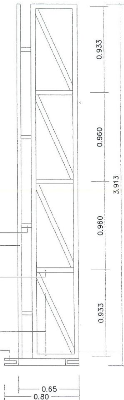
โครงเหล็กด้านข้าง
