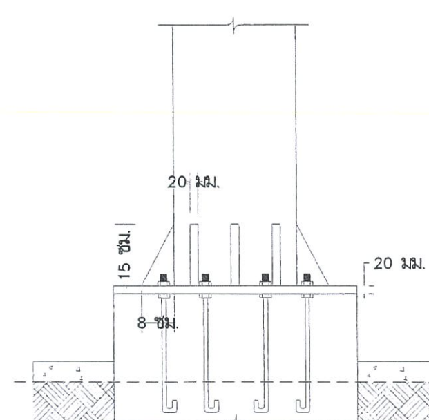
แปลนขยายเพลทฐาน
