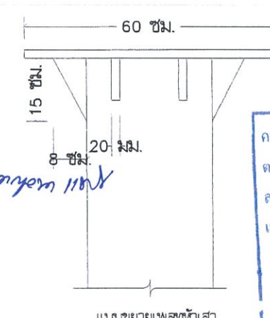
แปลนขยายเพลทหัวเสา
