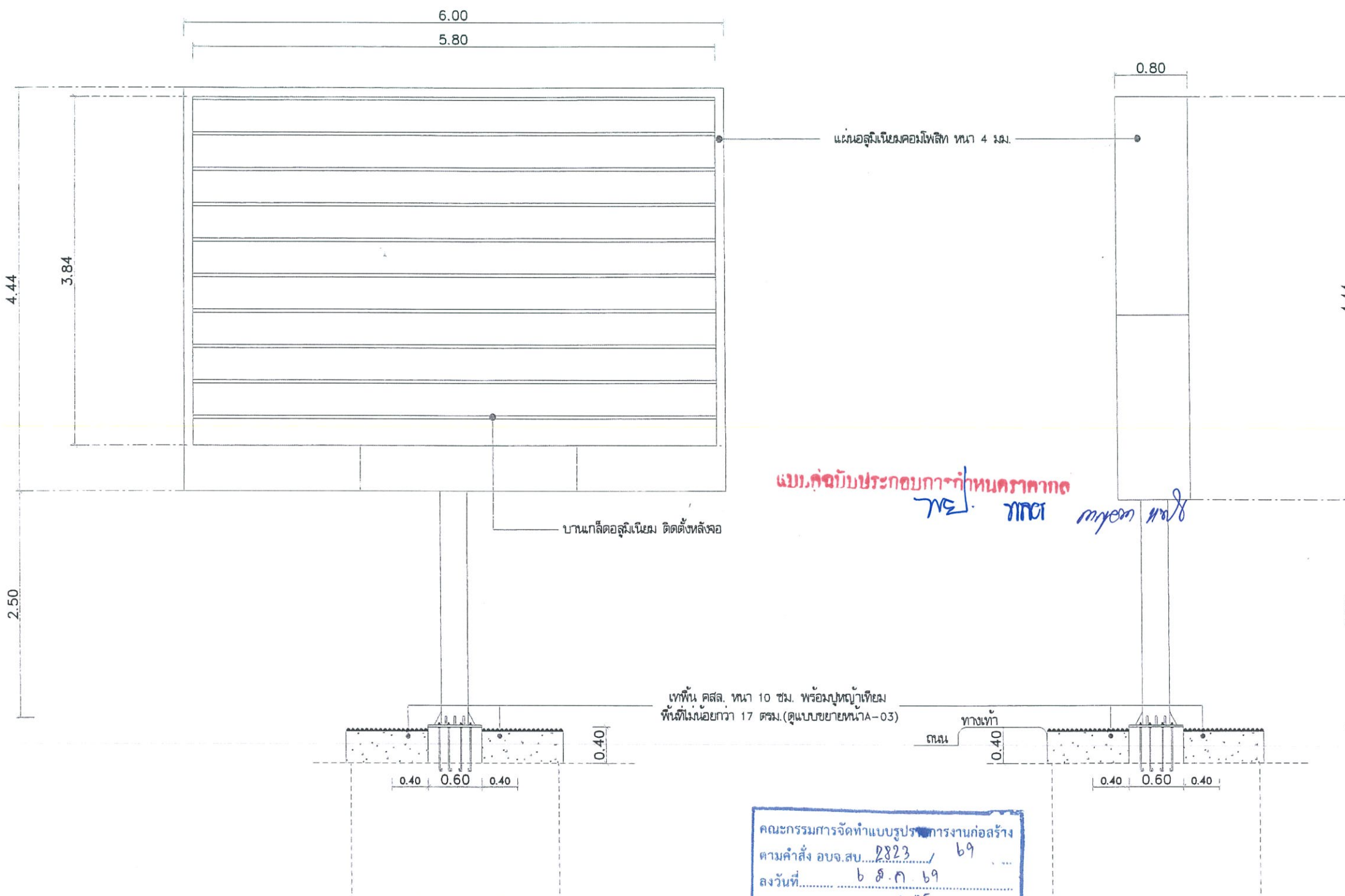
รูปด้านหลัง มาตราส่วน 1: 50
