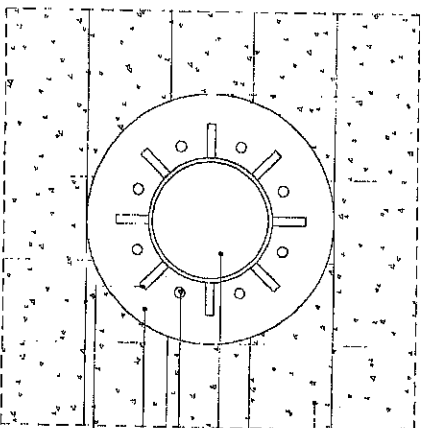
แบบขยายเหล็กเส้น
