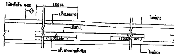
การตั้งเลนจราจร กรณีความกว้างของช่องจราจรลดลง
