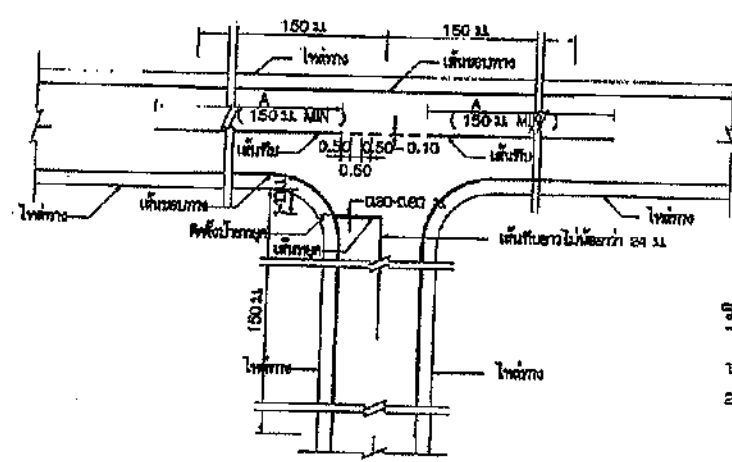
การตั้งเลนจราจรทางแยก
