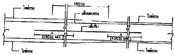
การตั้งเลนจราจร กรณีความกว้างของไหล่ทางลดลง
