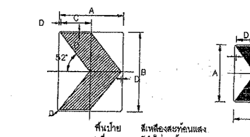
เว้นขอบป้าย สีเหลืองสะท้อนแสง เส้นขอบป้าย สีดำไม่สะท้อนแสง พื้นป้าย สีเหลืองสะท้อนแสง เครื่องหมาย สีดำไม่สะท้อนแสง
