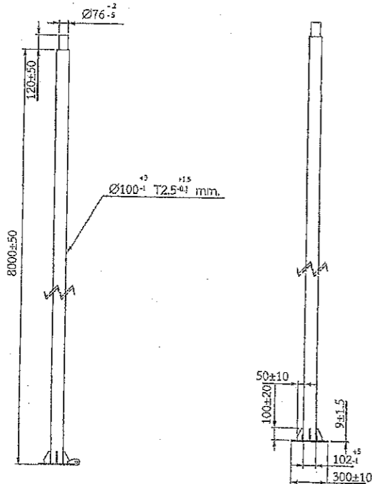
เสาไฟถนนประสงค์ แบบโคมเดียว หน่วย : มิลลิเมตร
