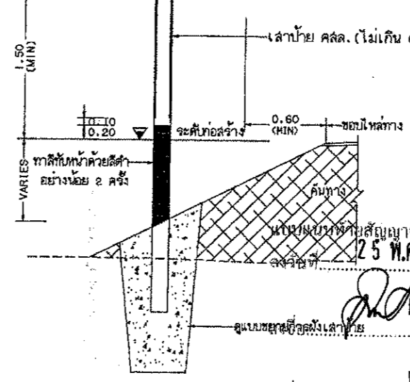
แสดงการปักเสาป้ายแนะนำ น-1 และ น-2
