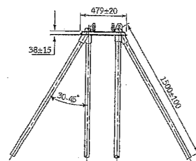
ฐานรากแบบหลายเข็ม (Multi-Pile Foundation) 3 แบบ บัญชีนวัตกรรมไทย 07020037 แบบ A ใช้กับพื้นที่ปกติ หน่วย : มิลลิเมตร
