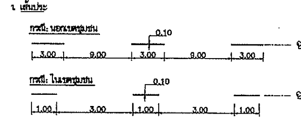
ขนาดและระยะของเครื่องหมายจรวดบริเวณผิวทาง
