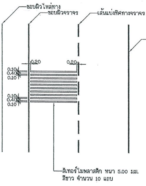
แบบขยาย RUMBLE STRIPS
