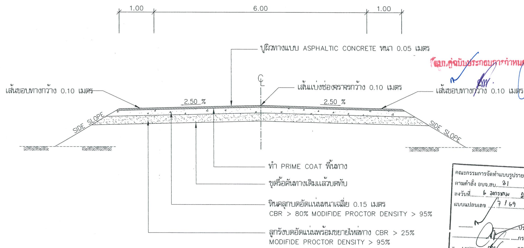
รูปตัดตามขวาง Asphaltic concrete
