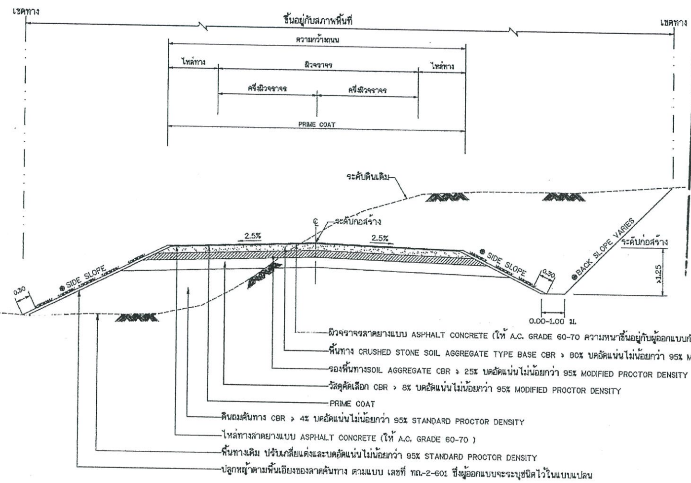
รูปตัดแสดงโครงสร้างถนนดินตัด ดินถมและคลุมสุมบ่อดีวีลวด
