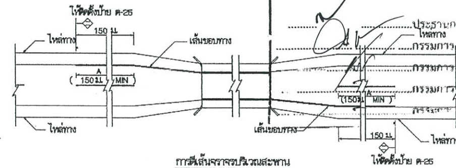
การติดตั้งจราจรบริเวณสะพาน
