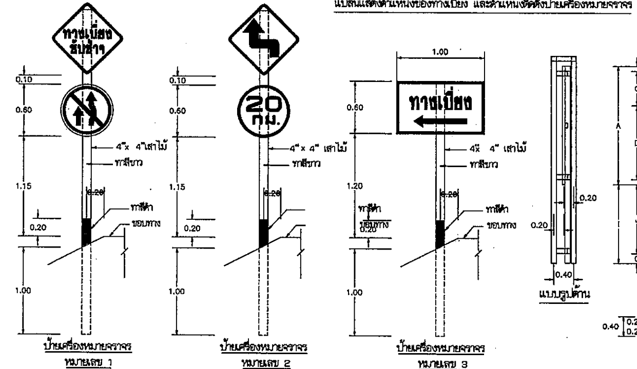
แปลนแสดงตำแหน่งของทางเบี่ยง และตำแหน่งติดตั้งป้ายเครื่องหมายจราจร
