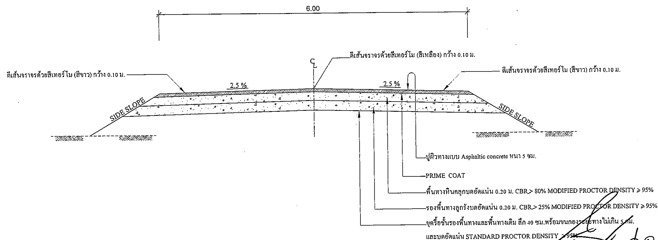
รูปตัดตามขวาง ASPHALT CONCRETE
