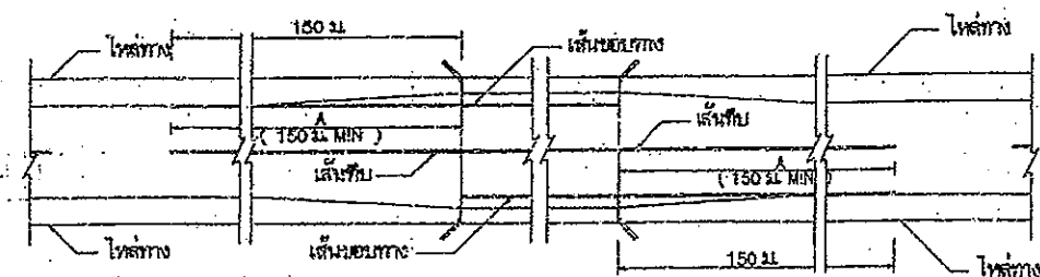
การให้ความกว้างสะพานน้อยกว่าความกว้างขี้นจระเข้ตาม
