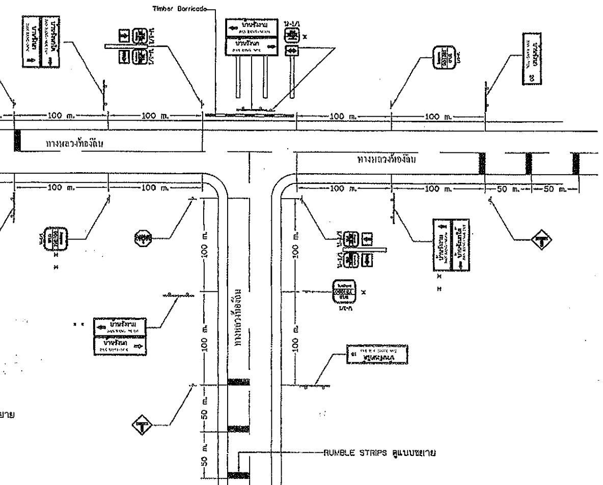
แสดงการติดตั้งป้ายจราจรบริเวณสามแยก ( เชื่อมทางหลวงท้องถิ่น )
