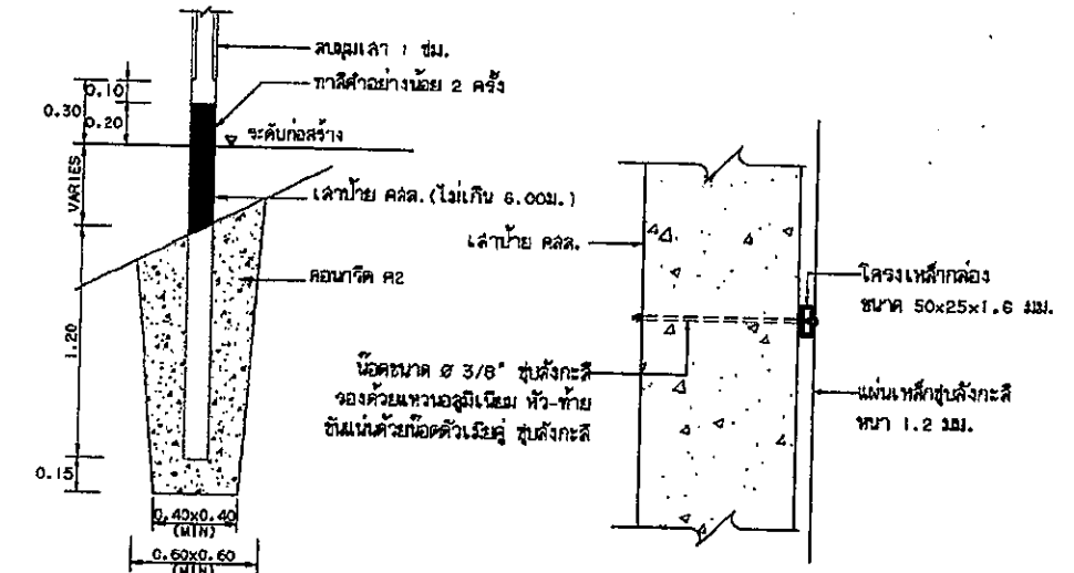
แสดงการติดตั้งเสาป้าย
