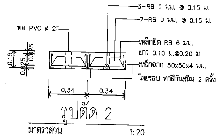
แปลนขยายเหล็กเสริมฝาบ่อพัก มาตราส่วน 1:20
