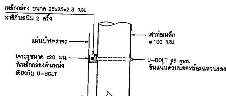
รูปตัด
