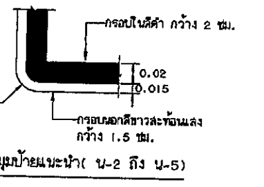
ป้ายหมายเลขทางหลวงท้องถิ่น น-2 (กรณีติดตั้งป้ายในเขตทางของทางหลวงท้องถิ่น) หน่วยเป็น เซนติเมตร
