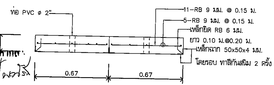
รูปตัด 2 มาตรฐาน 1:20
