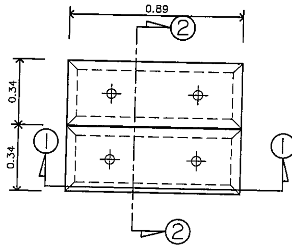
แปลนฝาบ่อพักในผิวจราจร มาตราส่วน 1:20
