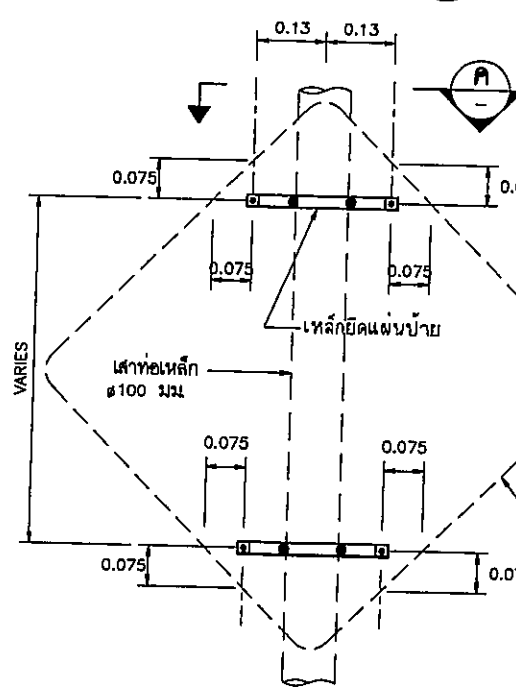
แบบขยาย "2" ไม่คงขนาดตัว
