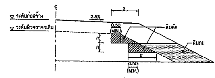
รูปตัดการก่อสร้างลาดดินทางบนถนนเดิม งานตัด ได้แก่ (งานตัดดิน, งานตัดหิน, งานตัดหินแข็ง และงานตัดอื่น ๆ)
