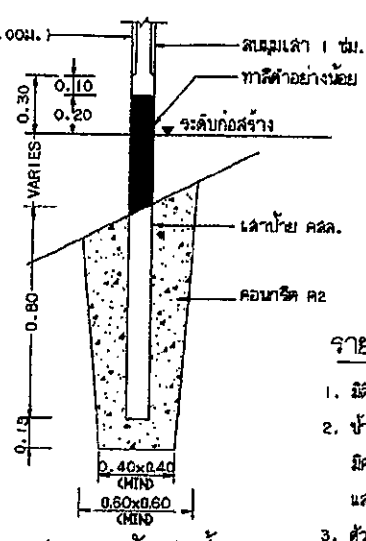
แสดงการปักเสาป้ายแนะนำ
