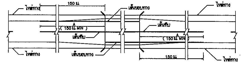
การเว้นระยะจากบริเวณโค้งรวม
