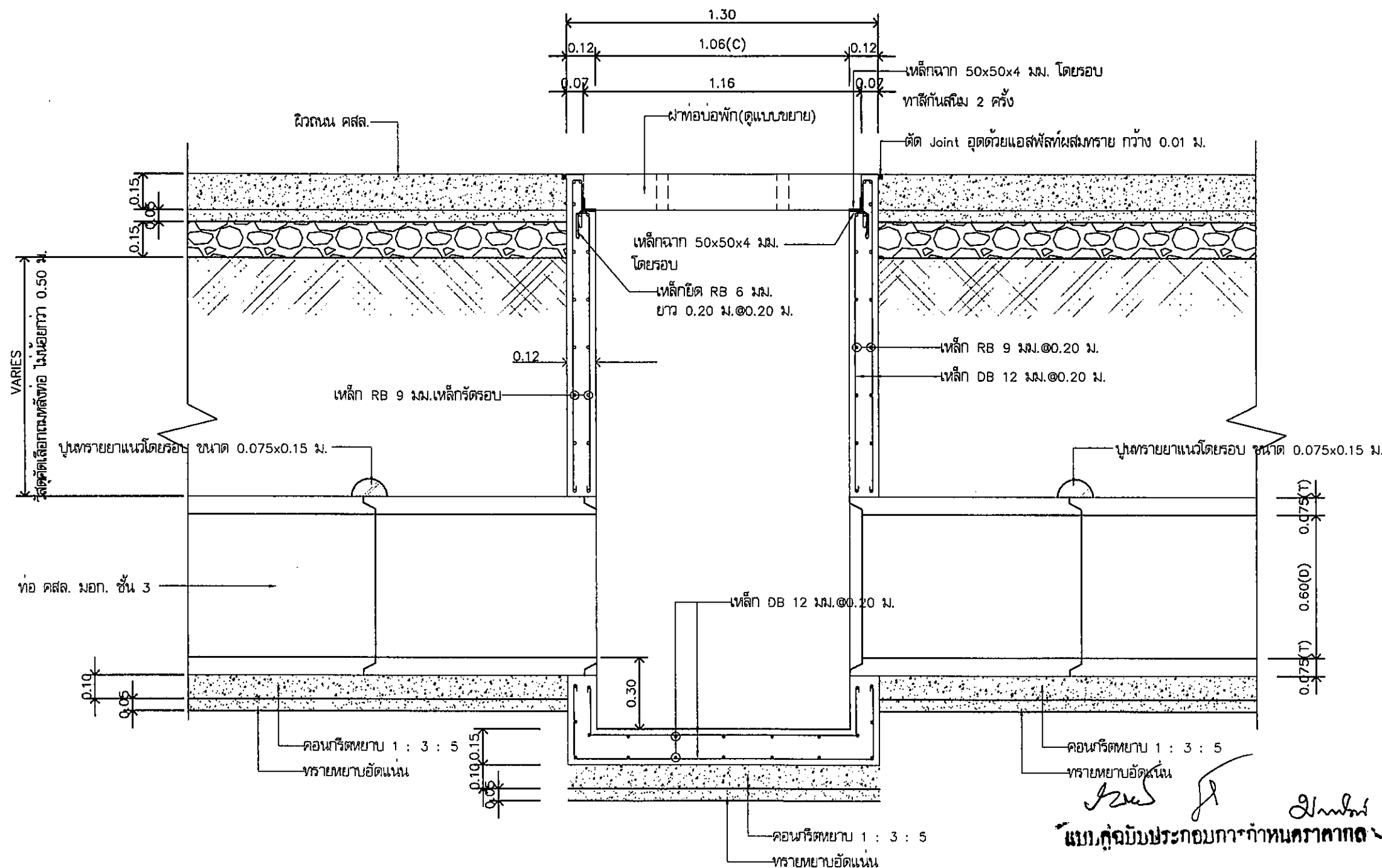
รูปตัดตามยาวท่อระบายน้ำในผิวจราจร ขนาด ๑๐.๖๐ ม. มาตรฐาน 1:20
