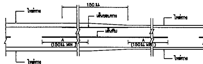
การเว้นระยะจากบริเวณโค้งรวม
