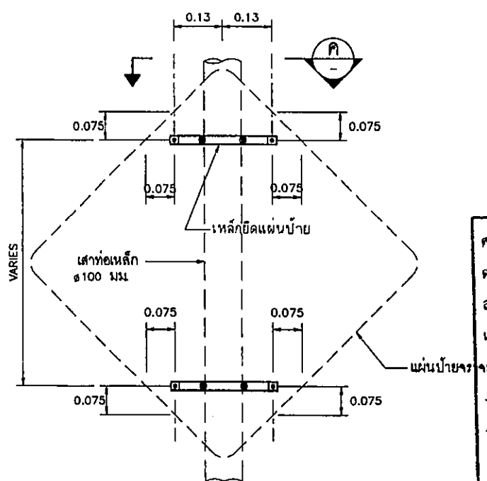
แบบขยายฐานจาก ไม่แสดงมาตราส่วน
