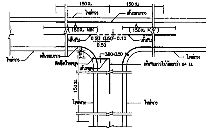
การเว้นระยะจากบริเวณโค้งรวม
