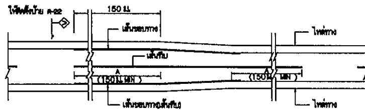
การเว้นระยะจากบริเวณโค้งรวม
