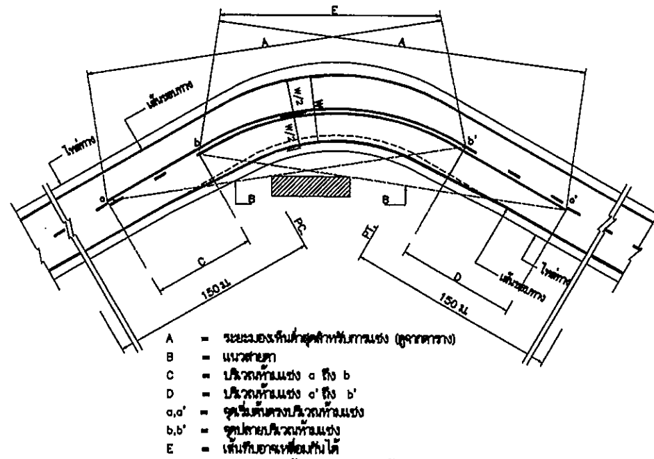
การตั้งเส้นจราจรบริเวณโค้งงา
