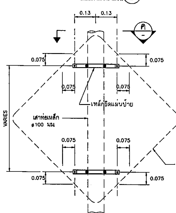
แบบขยายฐานจาก ไม่แสดงมาตราส่วน
