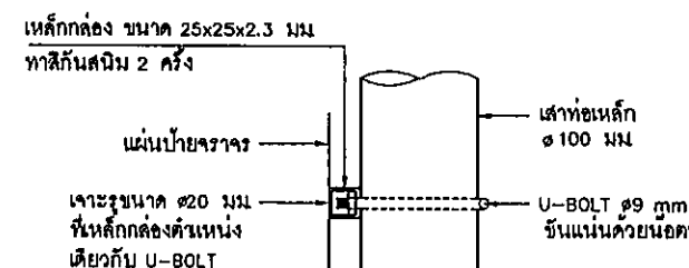
รูปตัด (จ) ไม่แสดงมาตราส่วน
