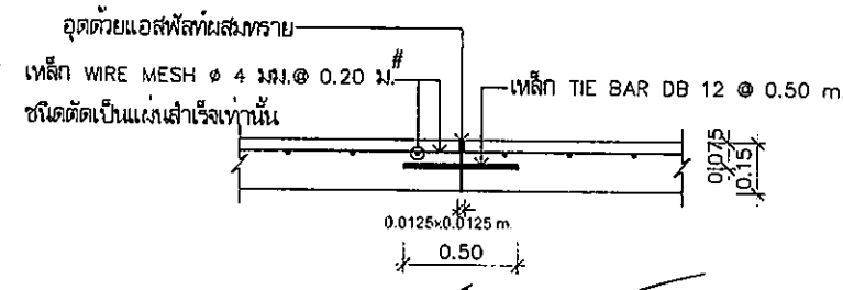
LONGITUDINAL JOINT
