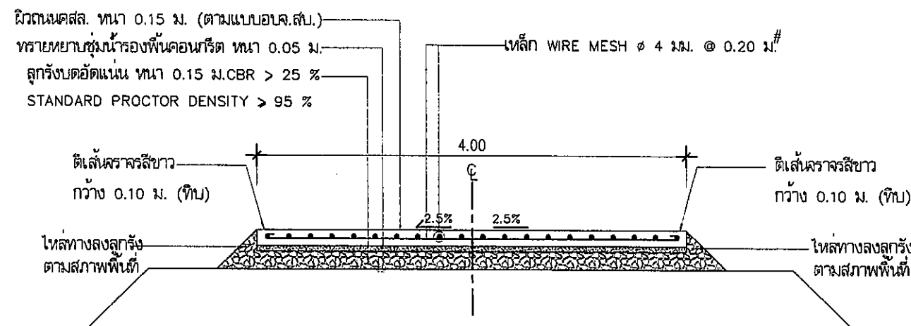
รูปตัดตามขวาง
