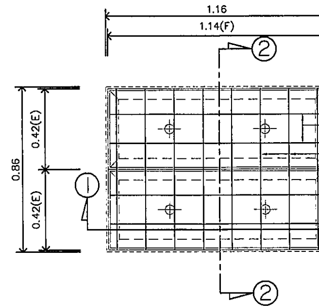
แปลนขยายเหล็กเสริมฝาบ่อพัก
