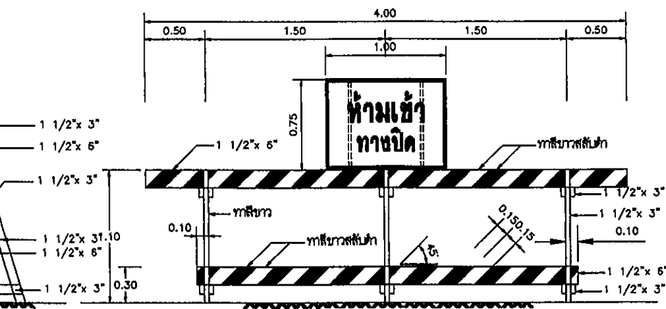
แปลนทำด้วยไม้ และป้ายเครื่องหมายจราจร หมายเลข 4
