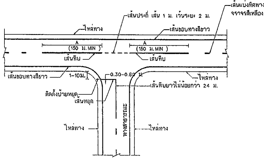
การตีเส้นจราจรทางแยก (ทางสามารณะ)
