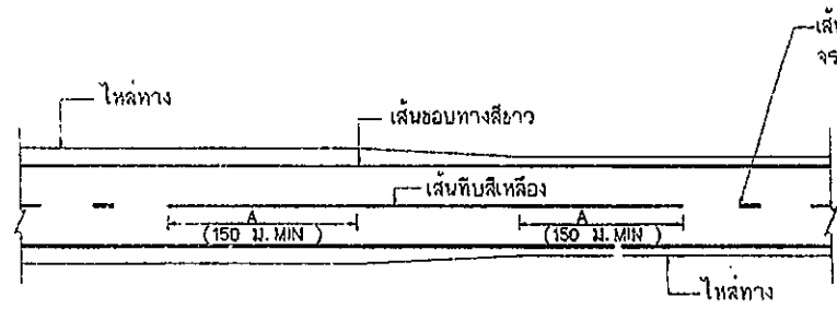
การตีเส้นจราจร กรณีความกว้างของไหล่ทางลดลง ไม่แสดงมาตราส่วน
