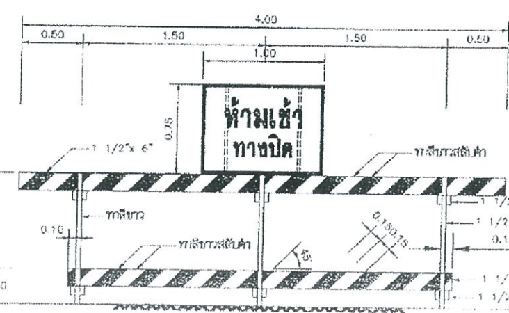
แผงกั้นด้วยไม้ และป้ายเครื่องหมายจราจร หมายเลข 4
