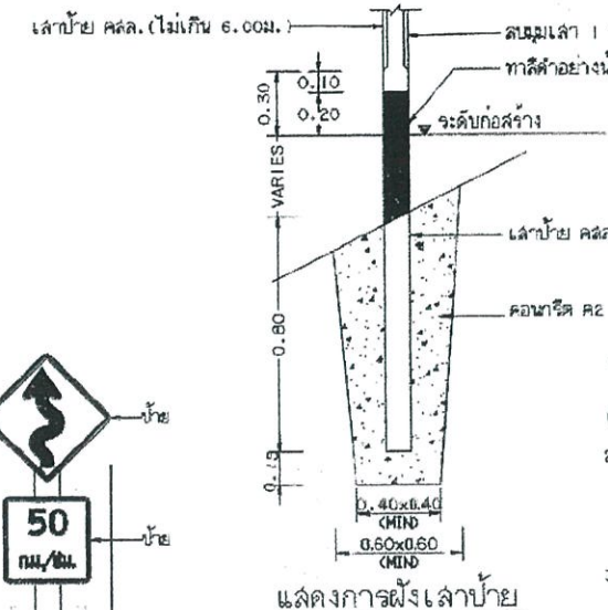
แสดงการปักเล้าป้ายบังคับและป้ายเตือน
