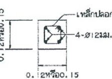
รูปตัด A-A
