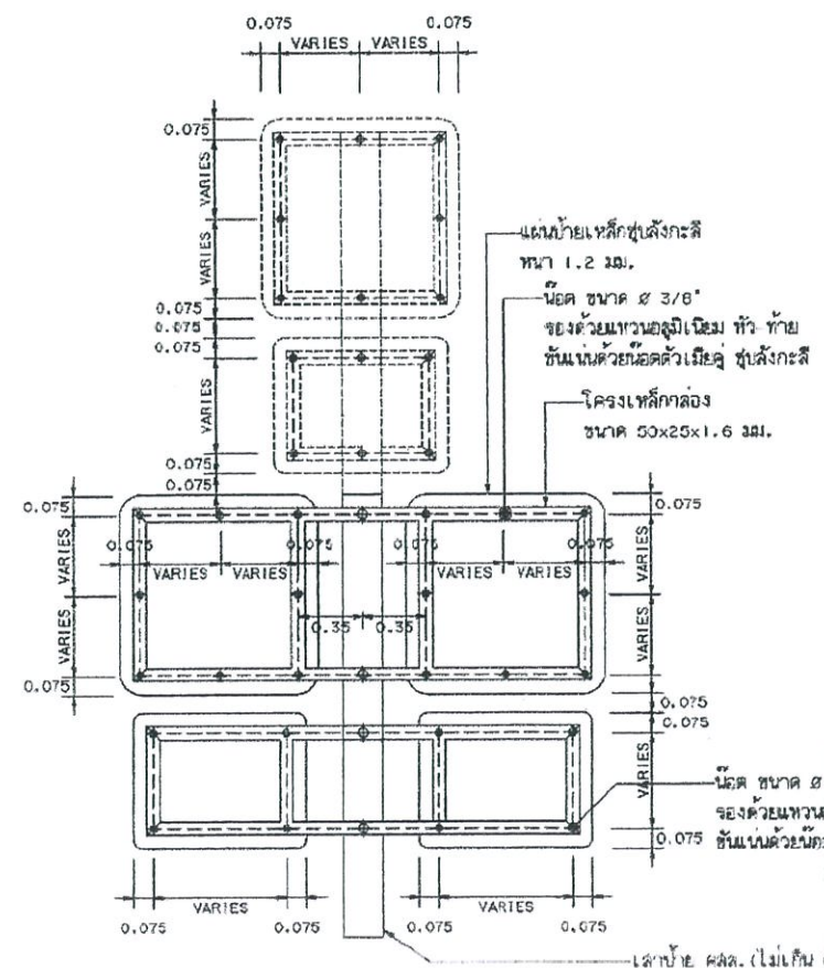
แสดงการยึดโครงป้ายชุดระบุทิศทาง
