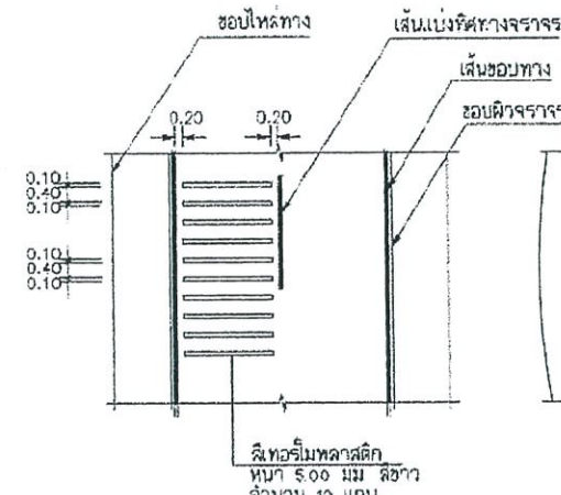
แบบขยาย A RUMBLE STRIPS
