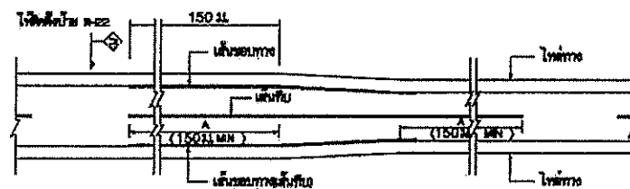
การเบี่ยงเบนจราจร กรณีความกว้างของช่องจราจรลดลง
