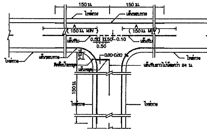
การเบี่ยงเบนจราจรทางแยก
