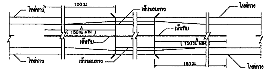
กรณีความกว้างช่องจราจรน้อยกว่าความกว้างผิวจราจรเลน
