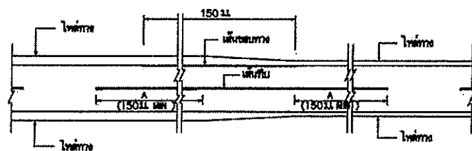
การเบี่ยงเบนจราจร กรณีความกว้างของเลนวิ่งลดลง
