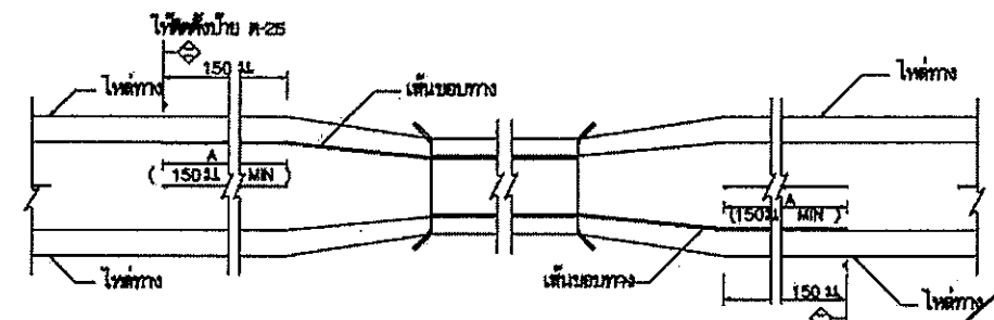
การเบี่ยงเบนจราจรบริเวณสะพาน
