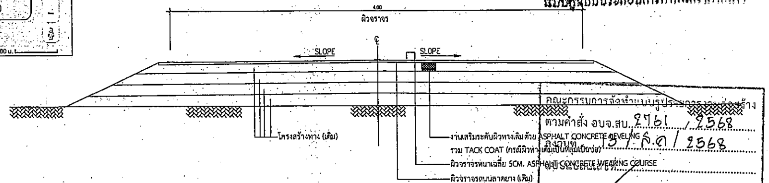
รูปตัดตามขวาง งานปรับปรุงผิวทาง ASPHALT HOT MIX OVERLAY
