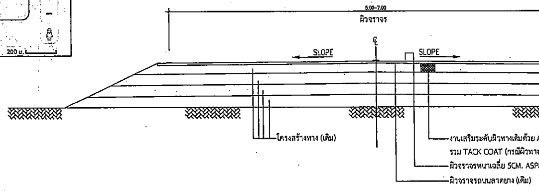
รูปตัดตามขวาง
