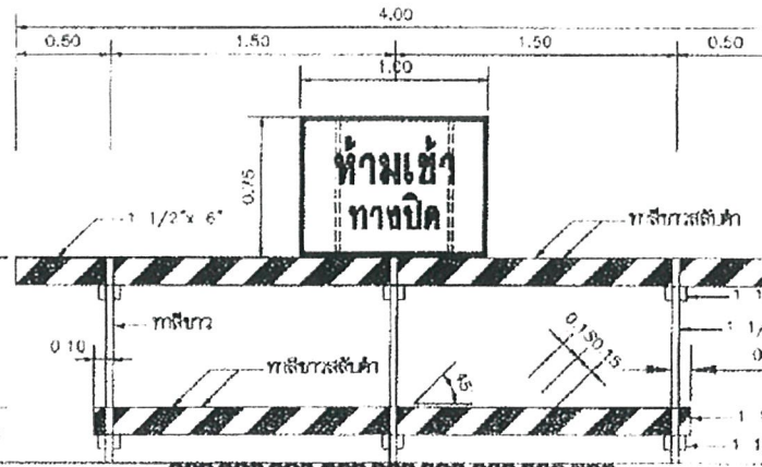
แผ่นป้ายด้วยไม้ และป้ายเครื่องหมายจราจร หมายเลข 4
