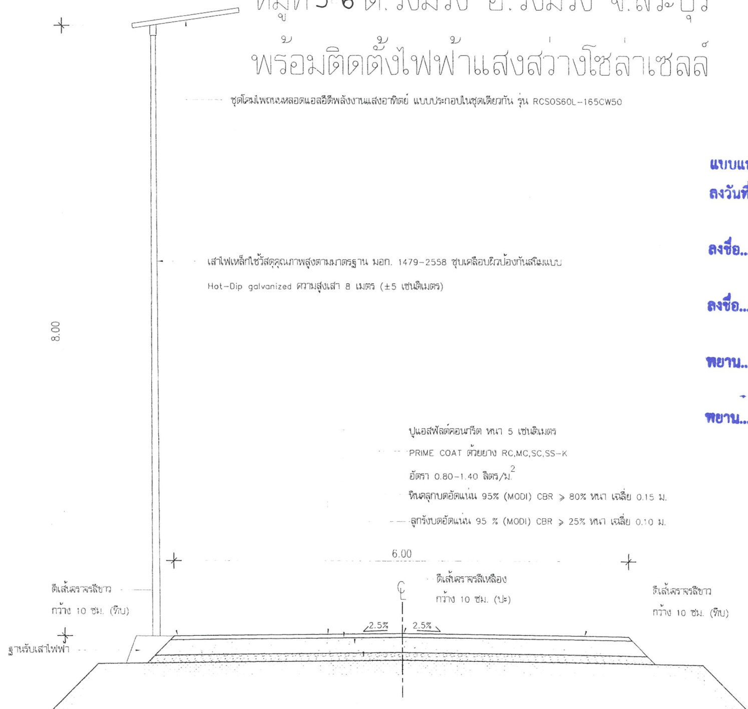
รูปตัดตามขวาง ก่อสร้างถนนลาดยางแบบแอสฟัลต์คอนกรีต (Asphalt Concrete)
