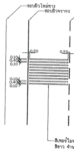
แบบขยาย RUMBLE STRIPS
