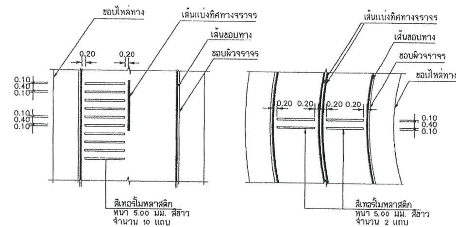
រំលង A RUMBLE STRIPS
