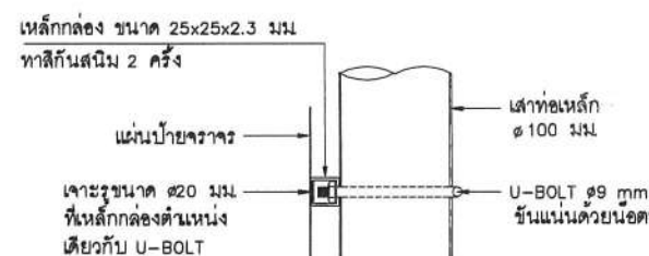
รูปตัด ไม่แสดงมาตราส่วน
