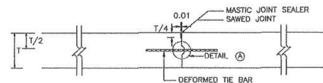
LONGITUDINAL JOINT
