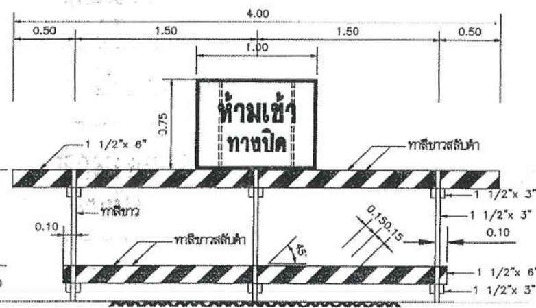
แพ่งกันทำด้วยไม้ และป้ายเครื่องหมายจราจร หมายเลข 4
