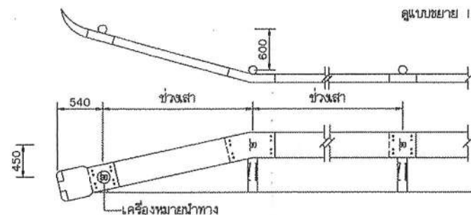
แบบขยาย 1. แล่งการติดตั้งและพับปลาย GUARD RAIL
