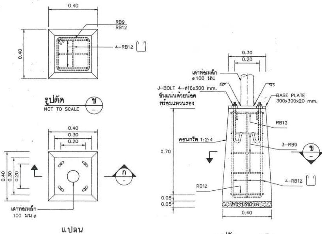
แสดงการติดตั้งสัญญาณไฟกระพริบร่วมกับป้ายบังคับหรือป้ายเตือน (เสาเหล็ก) ไม่แสดงมาตราส่วน
