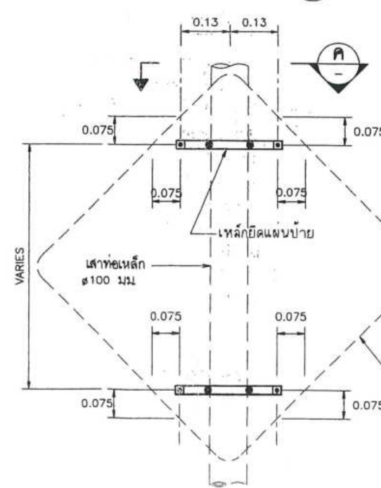
แบบขยาย "2"
