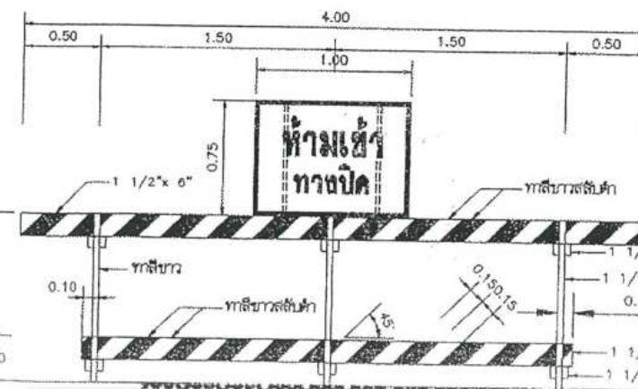
แปลนท้ายท้ายไม้ และป้ายเครื่องหมายจราจร หมายเลข 4
