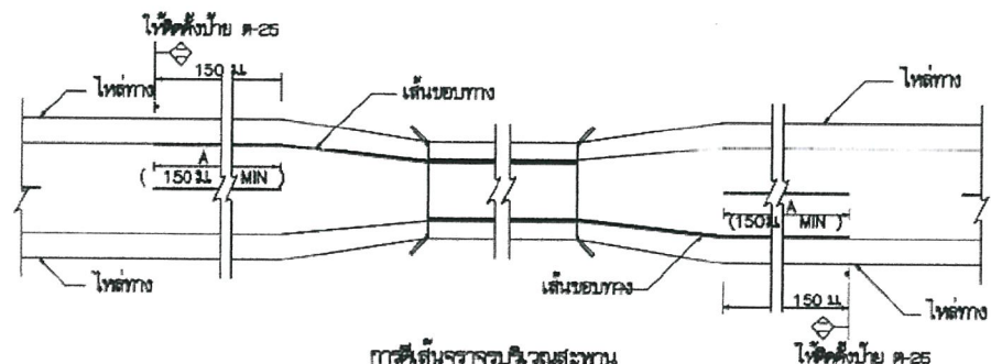
การเว้นระยะจากบริเวณสะพาน
