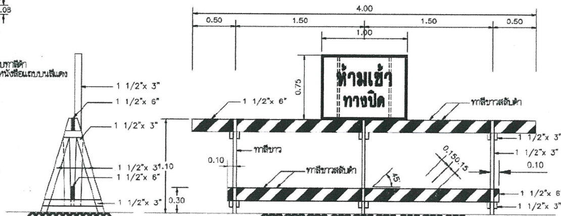
แปลนทำด้วยไม้ และป้ายเครื่องหมายจราจร หมายเลข 4
