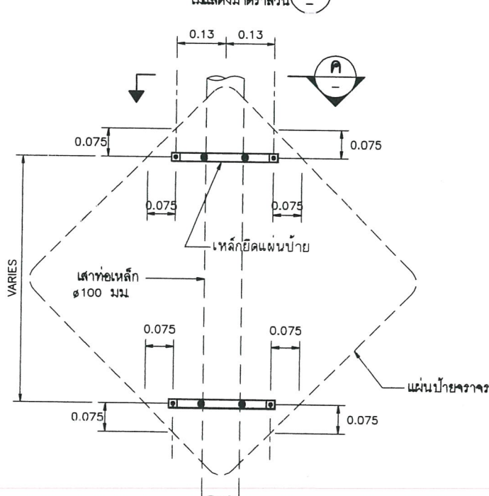
แบบขยายฐานราก ไม่แสดงมาตราส่วน
