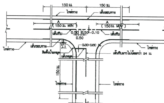
การเว้นระยะจากบริเวณแยก
