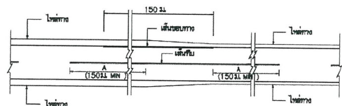
การเว้นระยะ การเว้นความกว้างของเลนวิ่งตลอด
