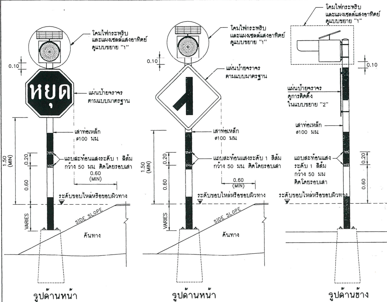
แสดงการติดตั้งสัญญาณไฟกระพริบร่วมกับป้ายบังคับหรือป้ายเตือน (เสาเหล็ก) ไม่แสดงมาตรฐาน
