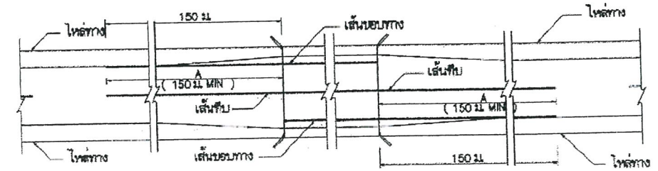
กรณีความกว้างช่องจราจรมากกว่าความกว้างผิวจราจรบน
