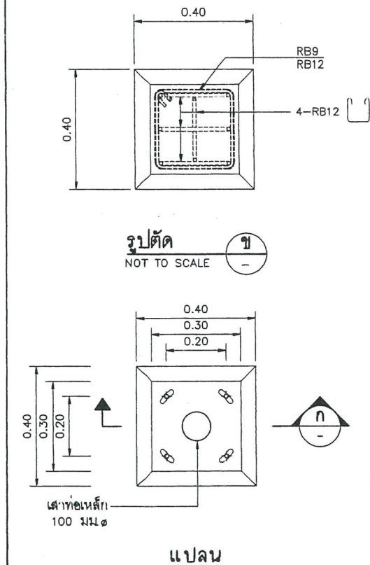
แสดงการติดตั้งสัญญาณไฟกระพริบร่วมกับป้ายบังคับหรือป้ายเตือน (เสาเหล็ก) ไม่แสดงมาตรฐาน
