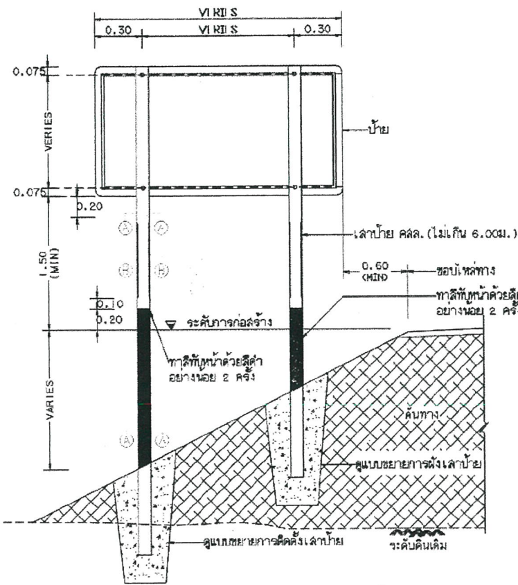
แสดงการปักเล้าป้ายแนะนำ น-2 น-3 และ น-4
