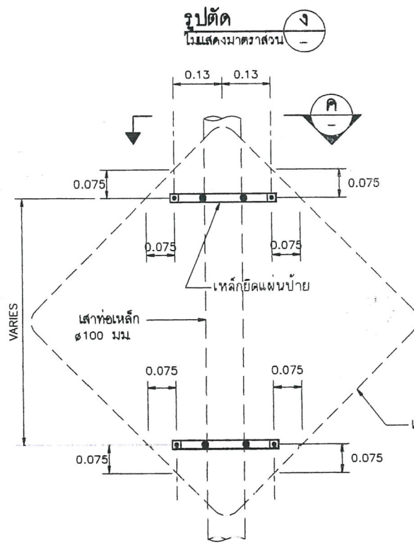
แบบขยาย "2" ไม่แสดงมาตรฐาน
