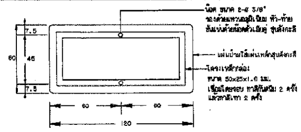
แสดงการยึดโครงป้ายโครงกรง น-1
