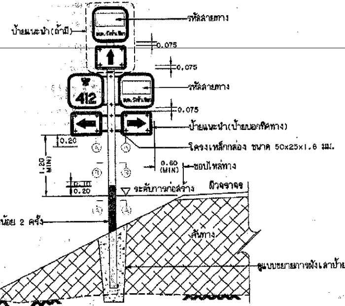
แสดงการติดตั้งเสาป้ายชุดระนาบทิศทาง
