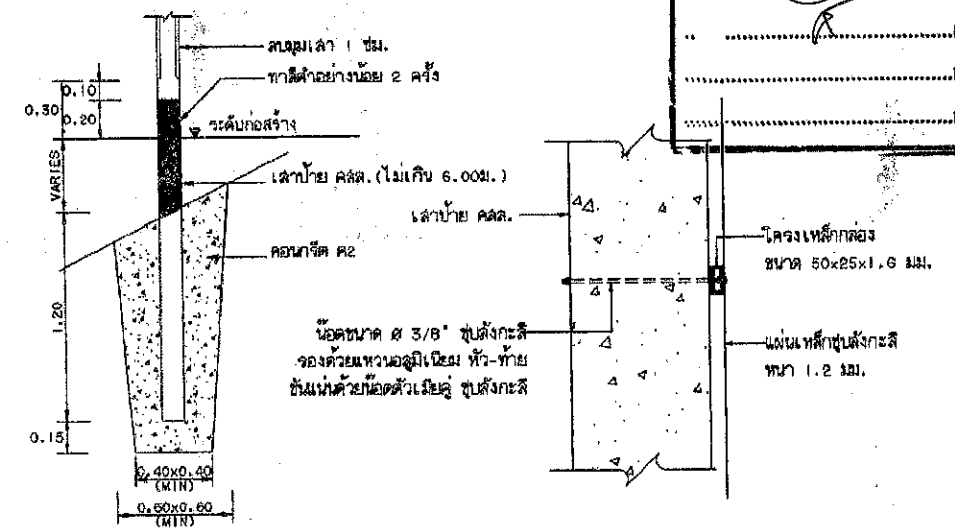
แสดงการฝังเสาป้าย รูปด้านข้างแสดงการยึดโครงป้ายกับเสา
