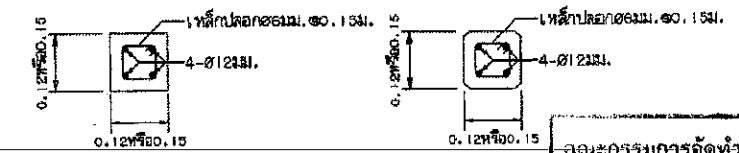
รูปตัด A-A (ดูหมายเหตุ ข้อ 4) รูปตัด B-B
