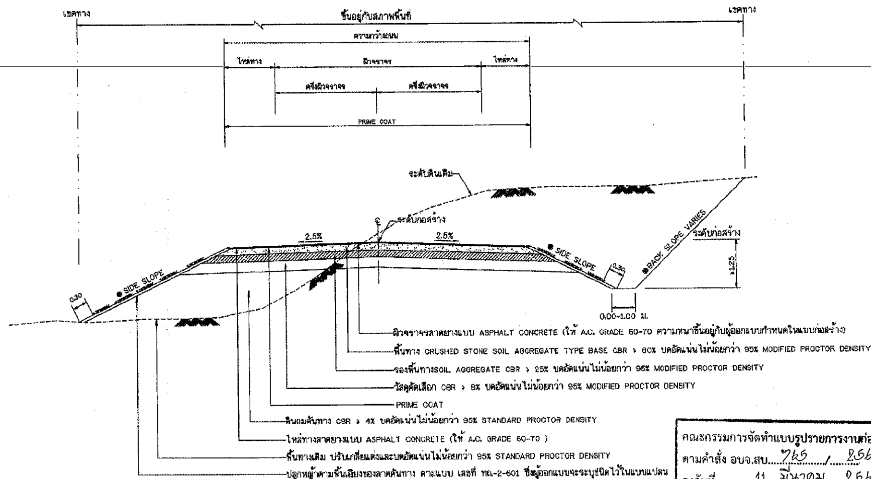
รูปตัดแสดงโครงสร้างถนนดินตัด ดินถมและคลุมสมบัติวัสดุ
