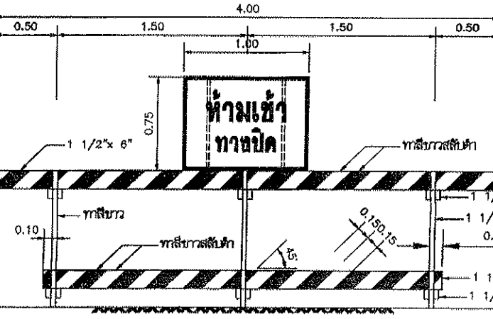
แผ่นกั้นทำด้วยไม้ และป้ายเครื่องหมายจราจร หมายเลข 4
