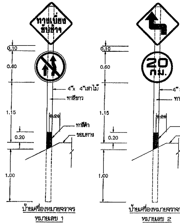
แบบแสดงตำแหน่งของทางเบี่ยง และตำแหน่งติดตั้งป้ายเครื่องหมายจราจร
