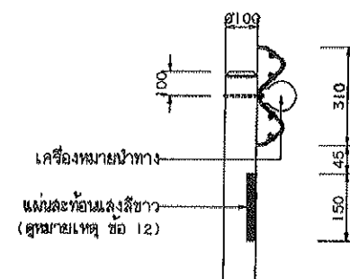
แบบแสดงเครื่องหมายนำทาง
