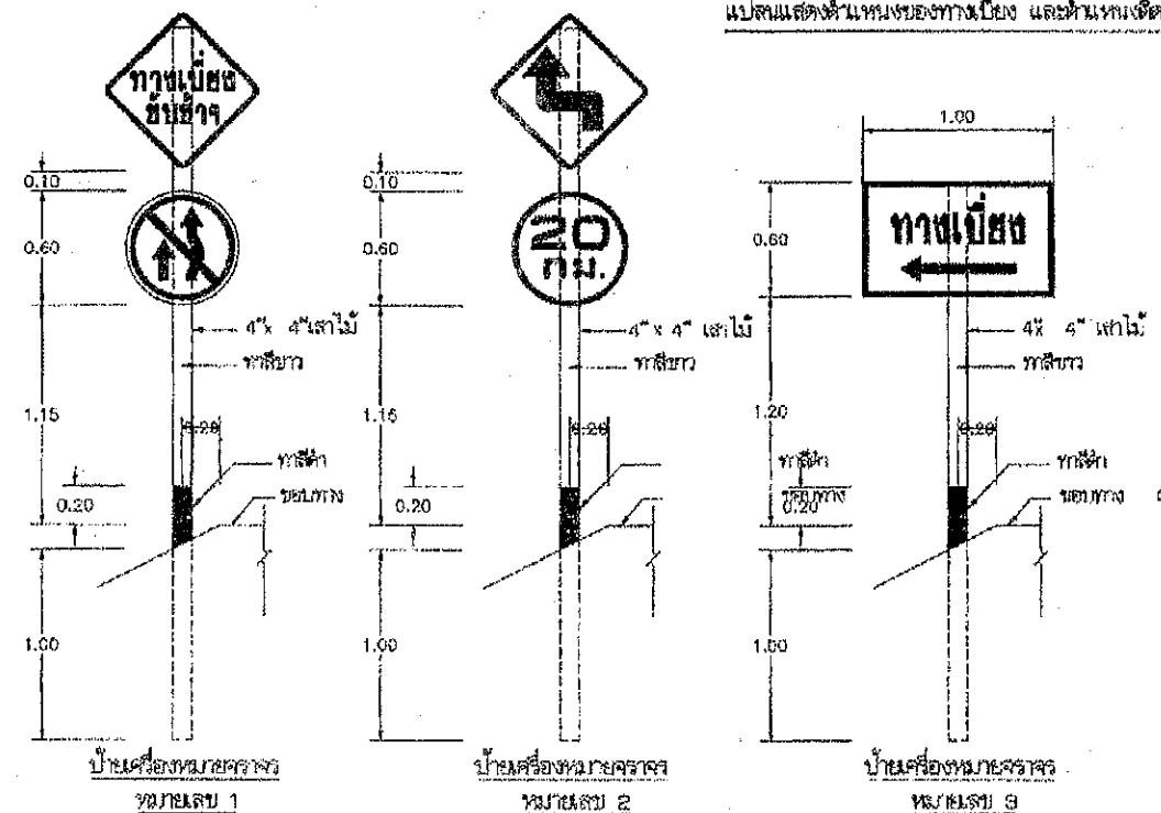
แบบแสดงตำแหน่งของทางเบี่ยง และตำแหน่งติดตั้งป้ายเครื่องหมายจราจร
