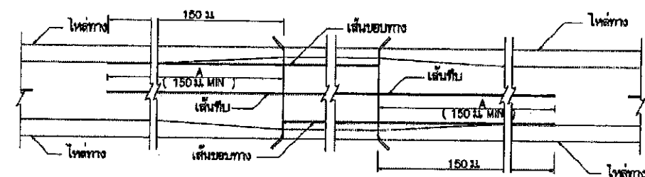
การให้ความกว้างสะพานน้อยกว่าความกว้างผิวจราจรถนน
