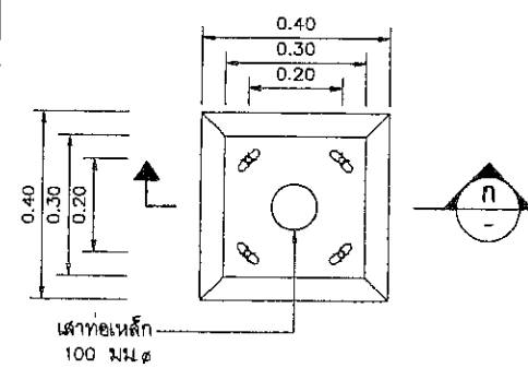
แปลน
