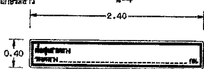
ป้ายสิ้นสุดสายทาง
