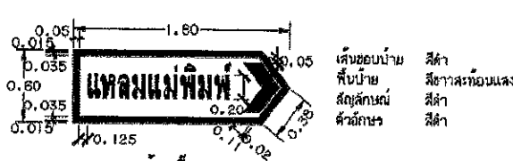
ป้ายชี้ทาง
