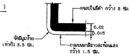
แสดงรูปป้ายแนะนำ (น-6 ถึง น-19)
