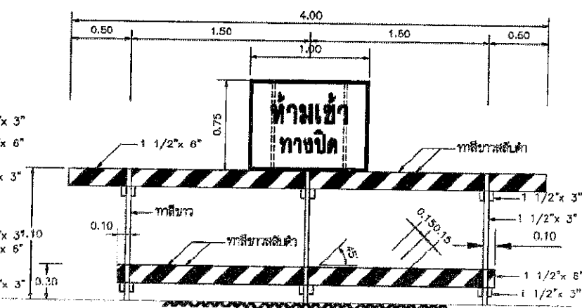
แผ่นที่ 71 ไม้ และป้ายจราจรจราจร หมายเลข 4
