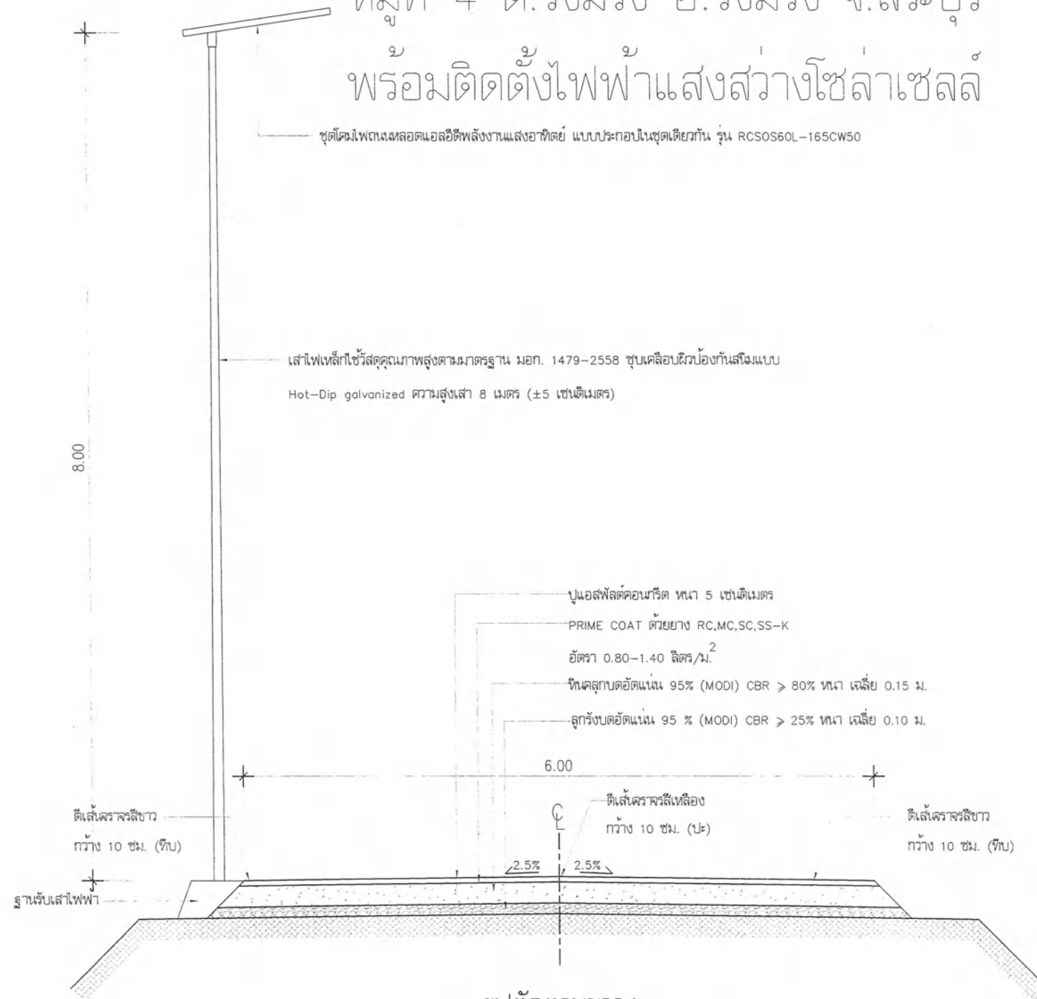
รูปตัดตามขวาง
