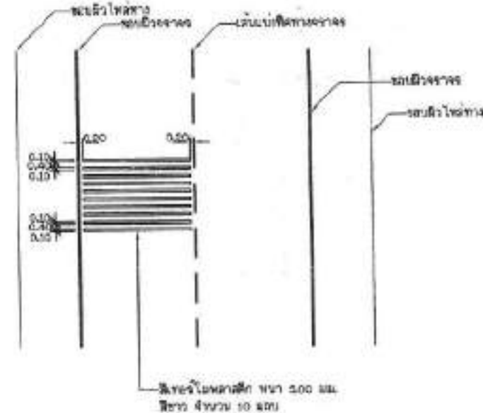
แบบขยี้ RUMBLE STRIPS
