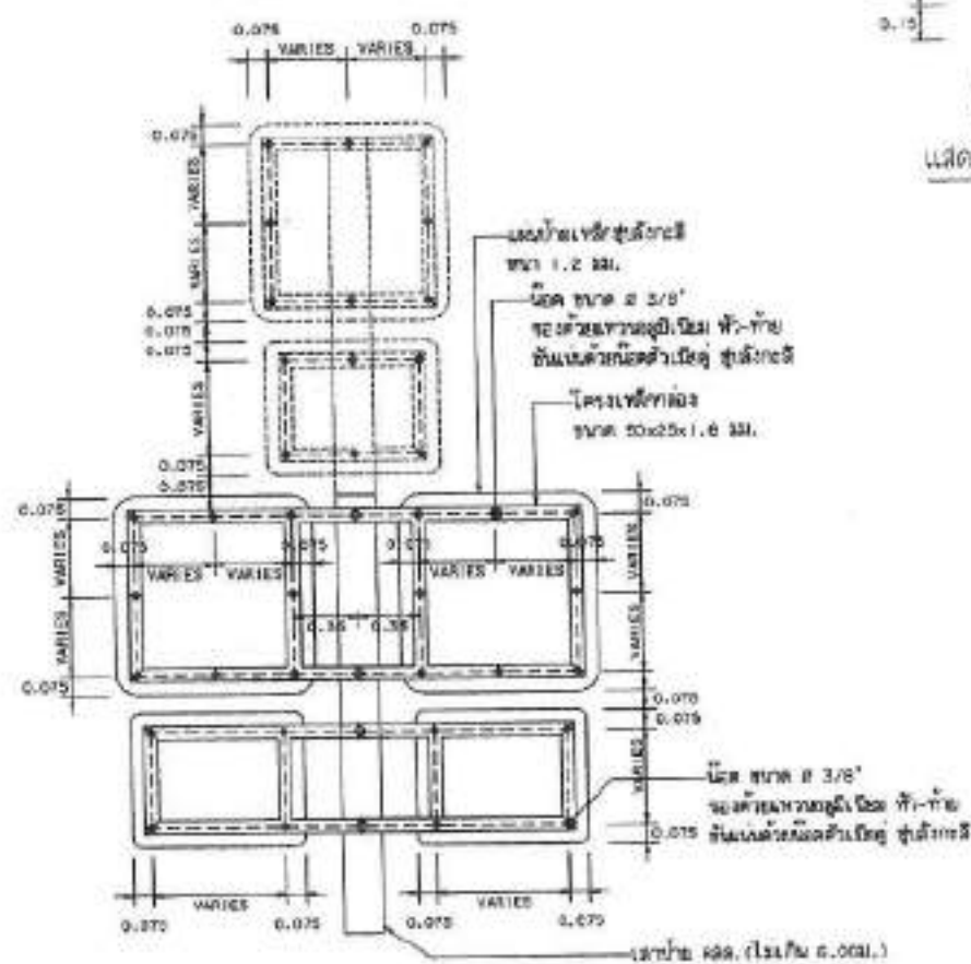
แสดงการติดตั้งเล้าป้ายชุดระบุทิศทาง
