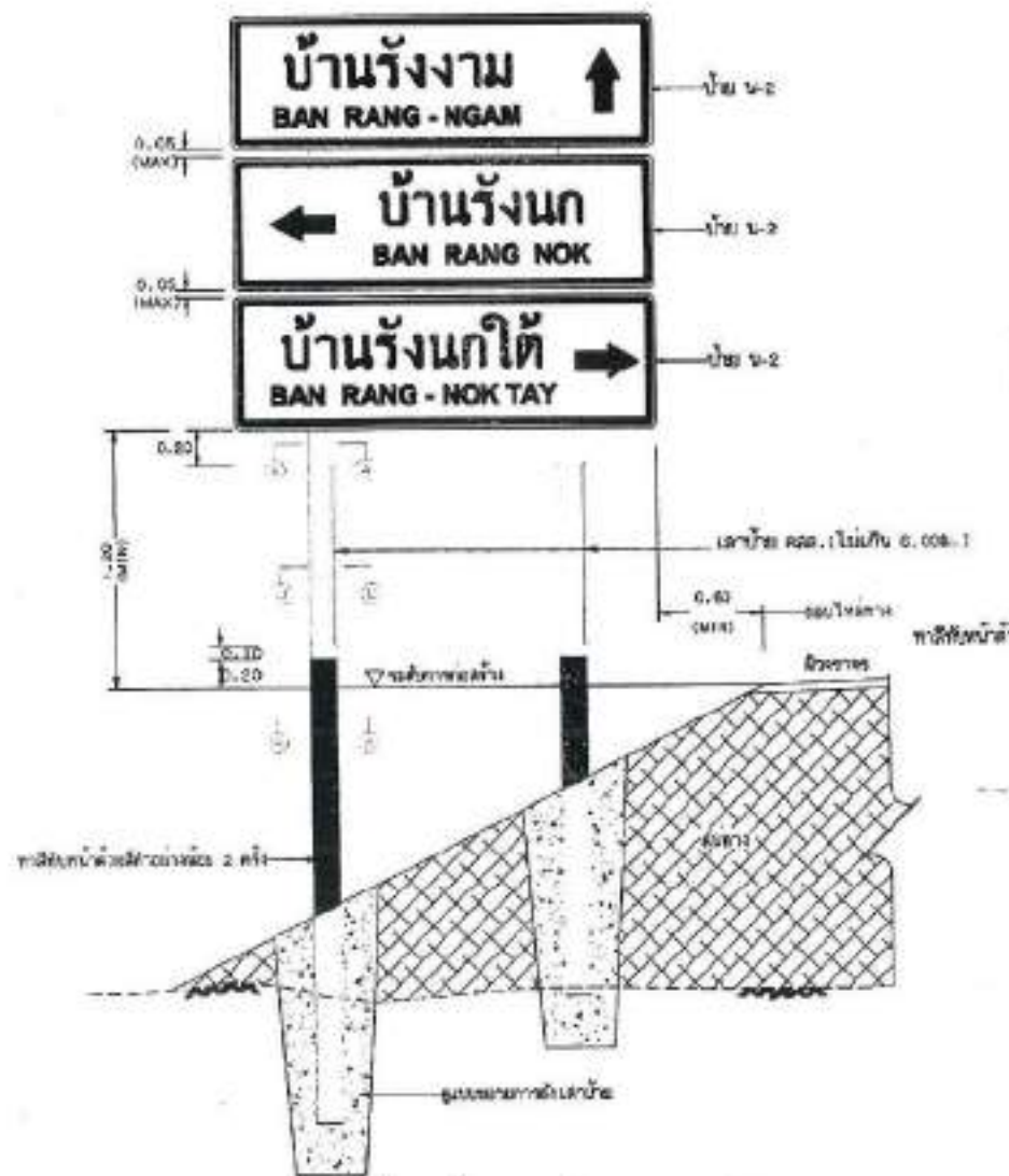
แสดงการติดตั้งเล้าป้าย น-2 (ชุด) และ น-3 (ชุด)
