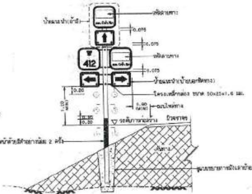
แสดงการติดตั้งเล้าป้ายชุดระบุทิศทาง
