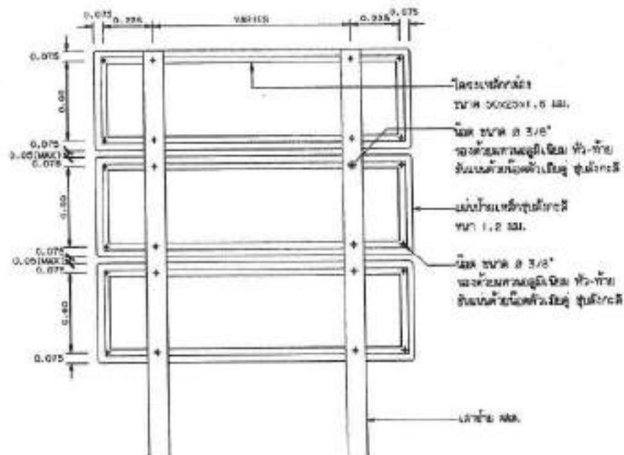
แสดงการติดตั้งเล้าป้าย น-2 (ชุด) และ น-3 (ชุด)
