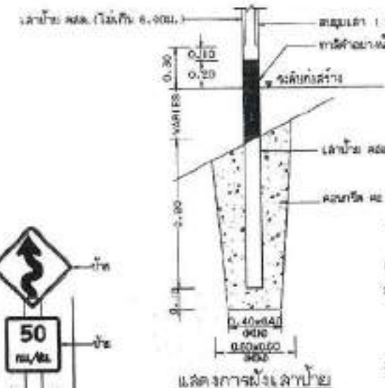
แสดงการปักเล้าป้ายแนะนำ น-4 และ น-6
