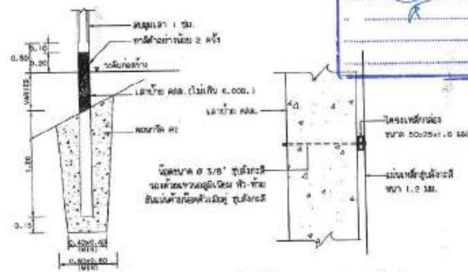
แสดงการติดตั้งเล้าป้าย
