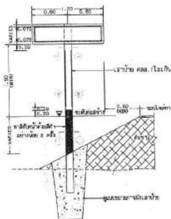
แสดงการปักเล้าป้ายแนะนำ น-4 และ น-6
