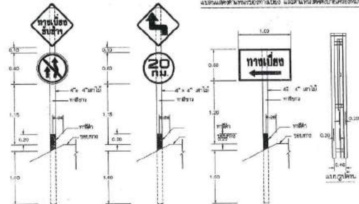
แบบแปลนหน้าทางเบี่ยงทางเบี่ยง และด้านหน้าตั้งขึ้นก่อนหรือภายหลังการ
