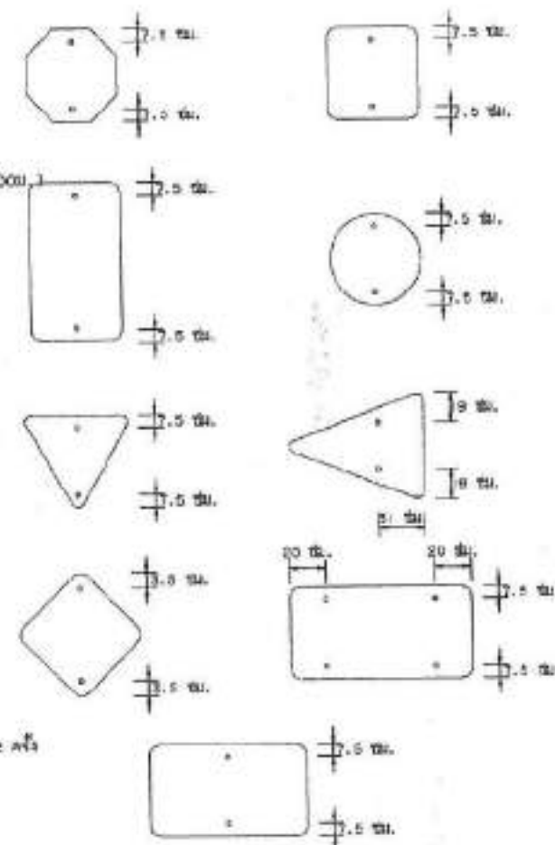
แสดงตำแหน่งการติดตั้งแผงป้ายบังคับ, ป้ายเตือน
