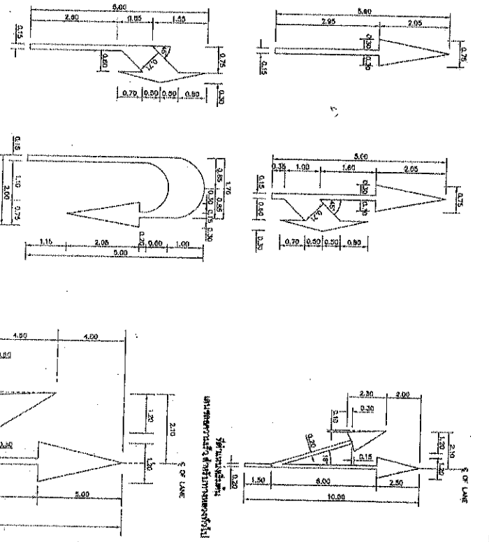
รูปแบบการขีดเส้นจราจร (DIRECTIONAL ARROWS)
