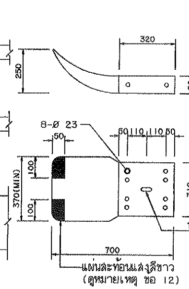
แบบแปลน GUARD RAIL
