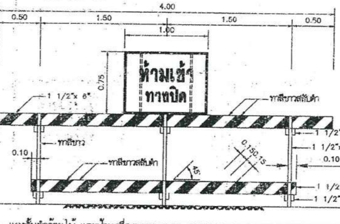
แผงกั้นที่ทำด้วยไม้ และป้ายเครื่องหมายจราจร หมายเลข 4
