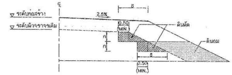
รูปตัดการก่อสร้างลาดคันทางบนถนนเดิม งานตัด ได้แก่ (งานตัดดิน, งานตัดหินหุ้, งานตัดหินแข็ง และงานกัดอื่น ๆ)
