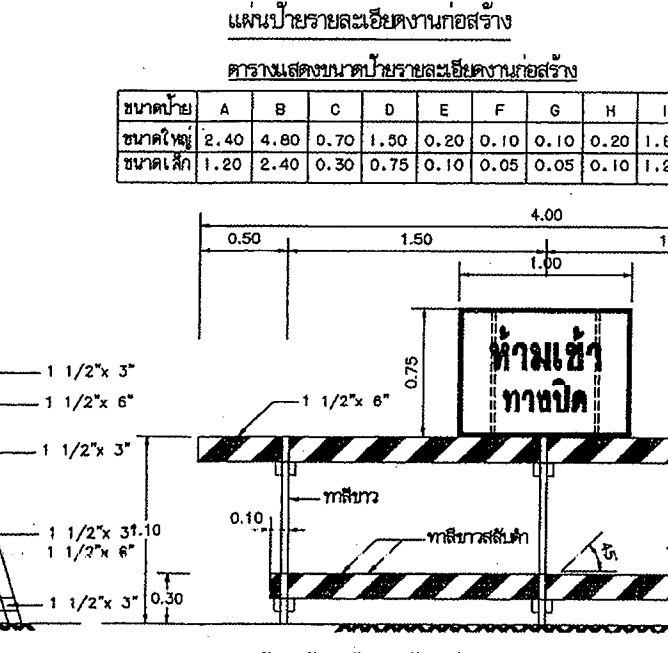
แผงกั้นทำด้วยไม้ และป้ายเครื่องหมายจราจร หมายเลข 4
