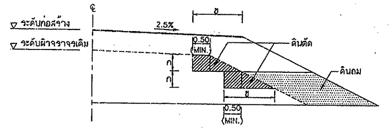
รูปตัดการก่อสร้างลาดคันทางบนถนนเดิม งานตัด ไถแก้ (งานตัดดิน, งานตัดหินหุ, งานตัดหินแข็ง และงานตัดอื่น ๆ)
