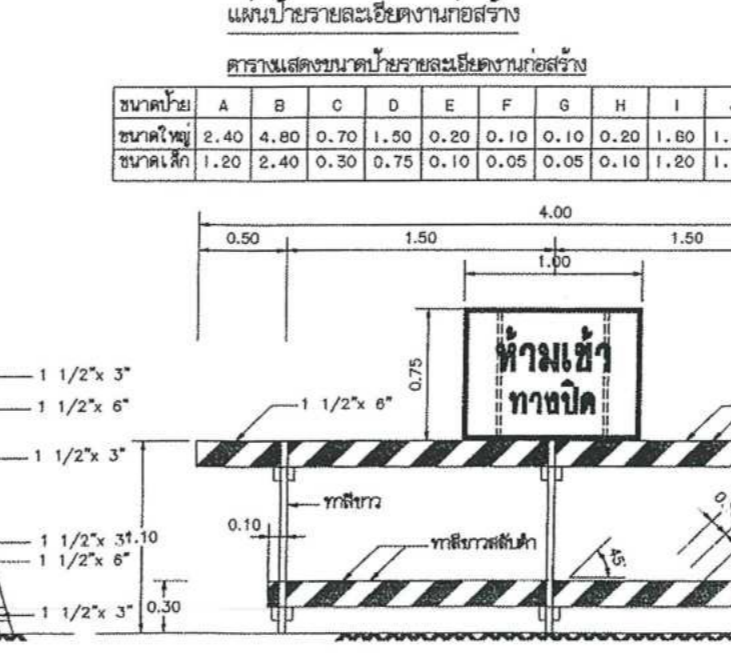
แผงกั้นทำด้วยไม้ และป้ายเครื่องหมายจราจร หมายเลข 4
