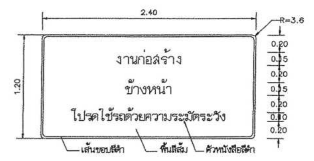
แบบก่อสร้างประกอบการทำหน้า
