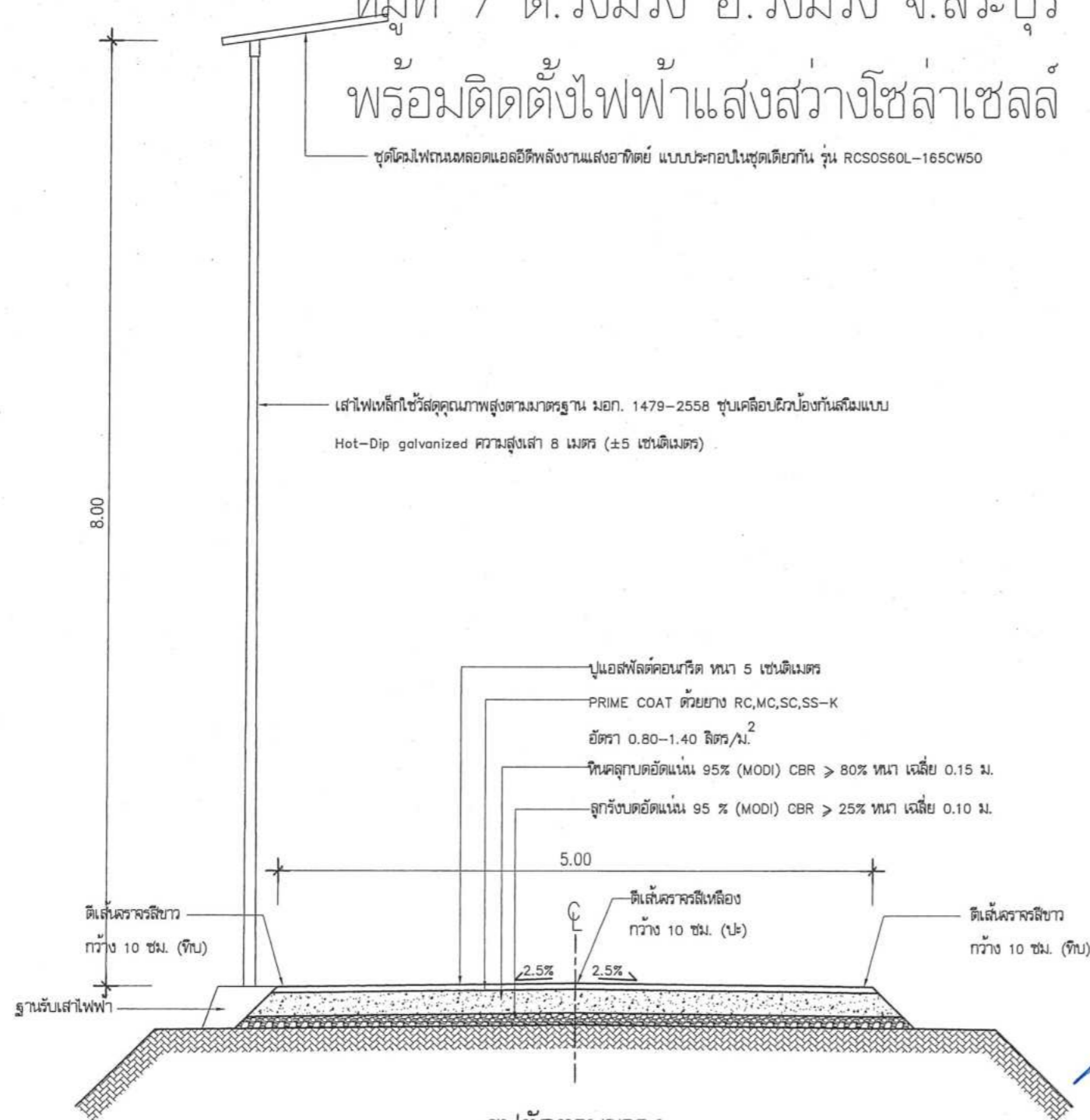
รูปตัดตามขวาง ก่อสร้างถนนลาดยางแบบแอสฟัลต์ติกคอนกรีต (Asphalt Concrete)
