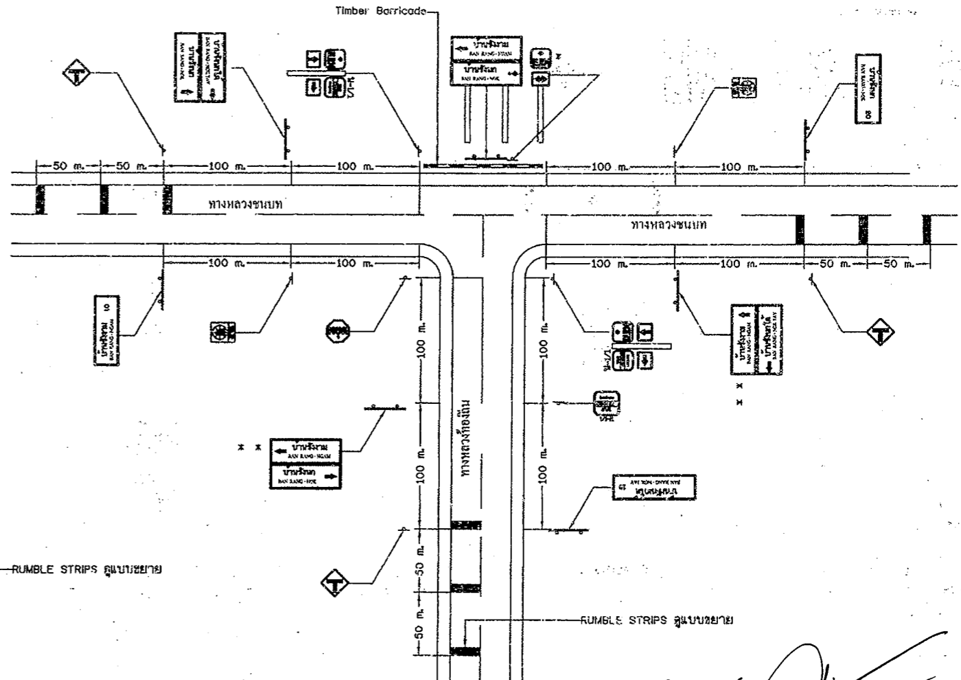
แสดงการติดตั้งป้ายจราจรบริเวณสามแยก ( เชื่อมทางหลวงชนบท ) แบบคู่ควมับประกอบกำหนดครากถนน
