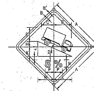
เว้นขอบบ้าย สีเหลืองสะท้อนแสง เส้นขอบบ้าย สีดำไม่สะท้อนแสง พื้นบ้าย สีเหลืองสะท้อนแสง เครื่องหมาย สีดำไม่สะท้อนแสง
