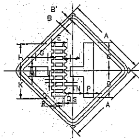
เว้นขอบบ้าย สีเหลืองสะท้อนแสง เส้นขอบบ้าย สีดำไม่สะท้อนแสง พื้นบ้าย สีเหลืองสะท้อนแสง เครื่องหมาย สีดำไม่สะท้อนแสง
