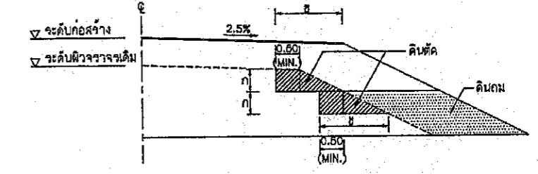
รูปตัดการก่อสร้างลาดคืนทางบนถนนเดิม งานตัด โคนัก (งานตัดดิน, งานตัดหินหุ่, งานตัดหินแข็ง และงานตัดอื่น ๆ)
