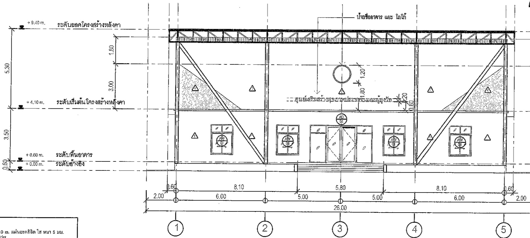
รูปด้าน 4
