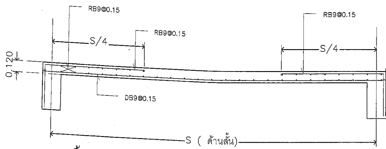
พื้น S2 SCALE 1:25 A3
