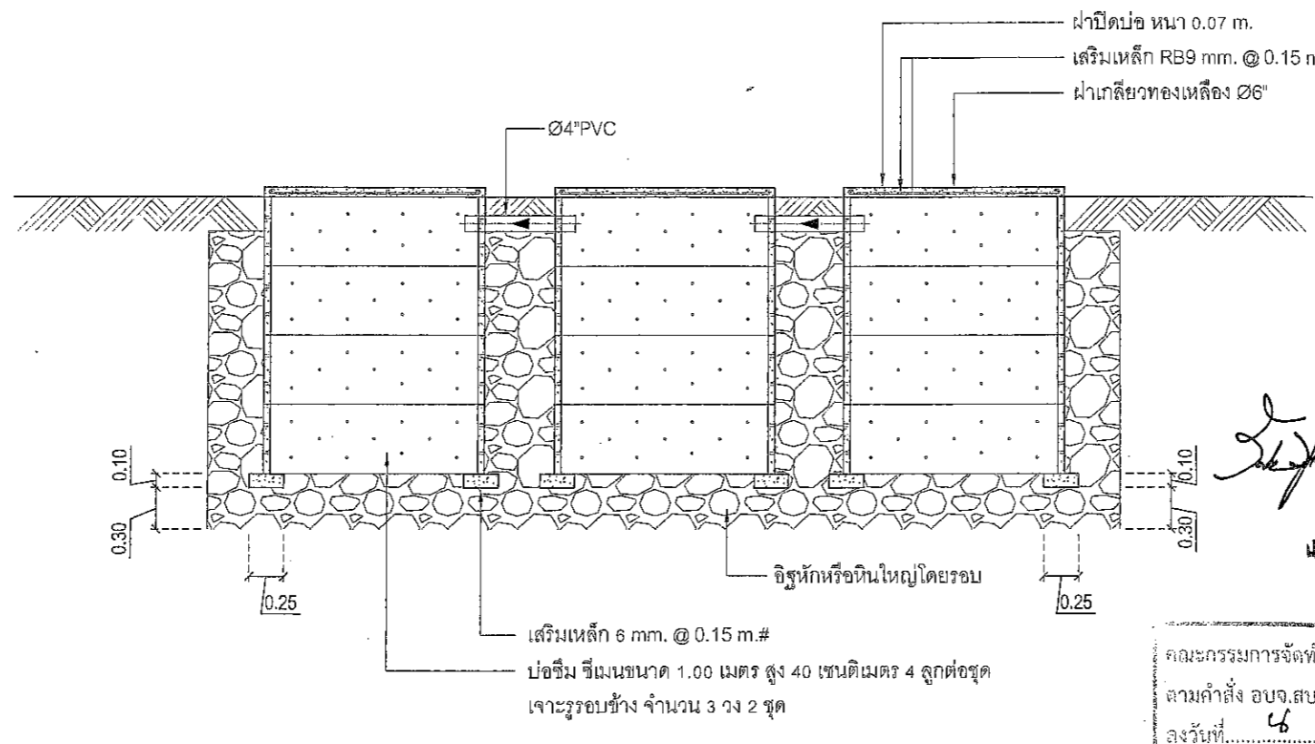
รูปตัดบ่อซึม
