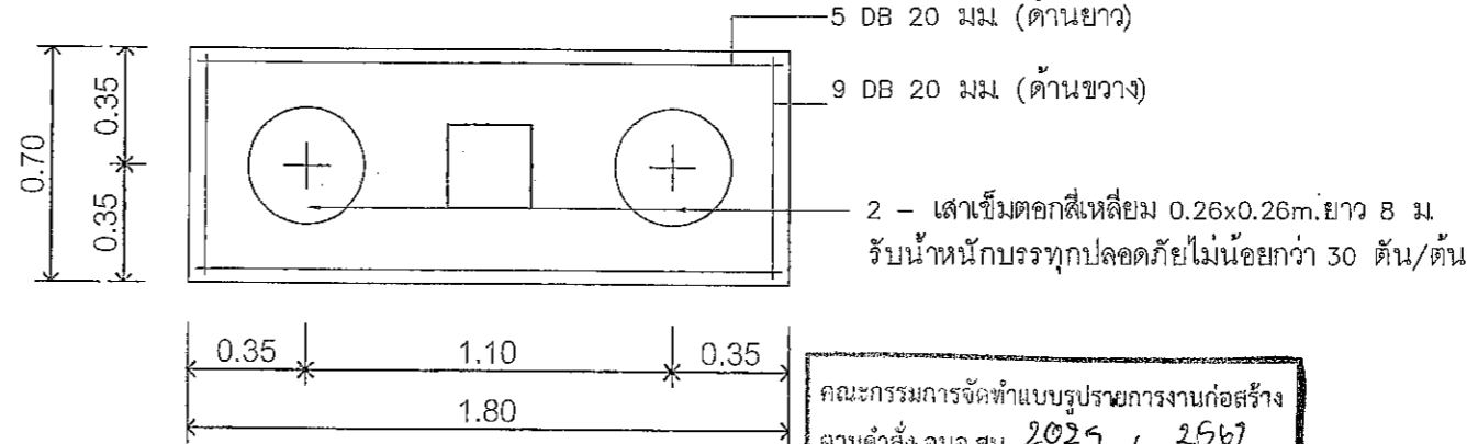
F2 แบบขยายฐานราก, ตอม่อ, เสาค้ำ SCALE 1:25
