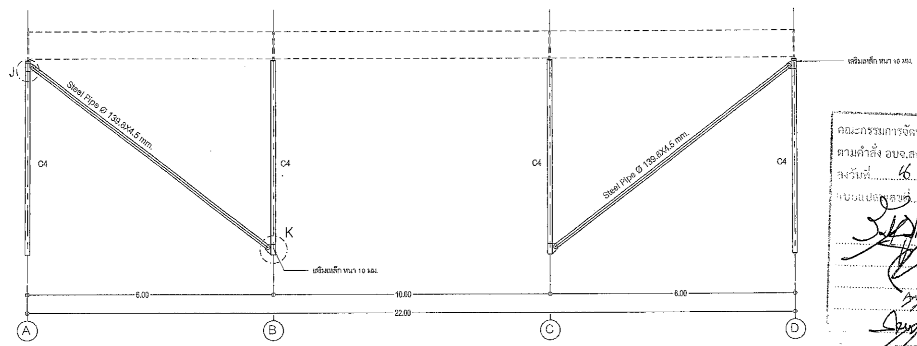
แบบขยาย FRONT STEEL PIPE SCALE 1:125 A3
