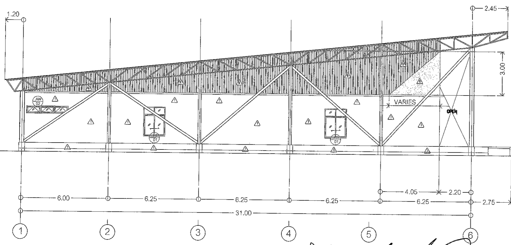
รูปด้าน 2 SCALE 1:150 A3
