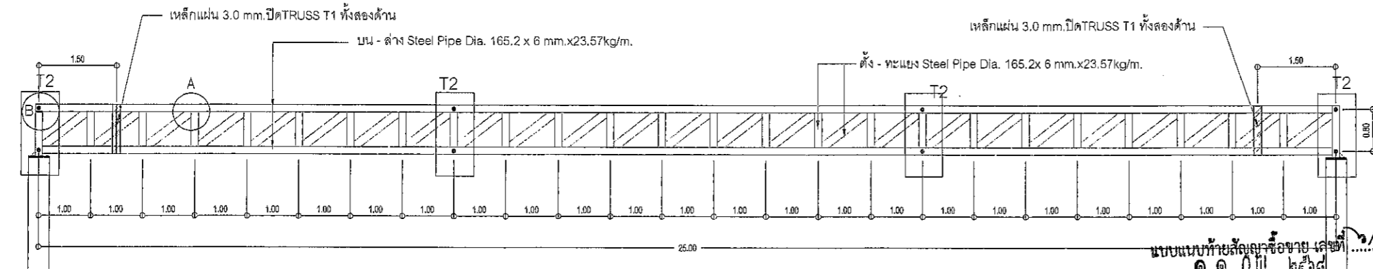
TRUSS T1 SCALE 1:100 A3
