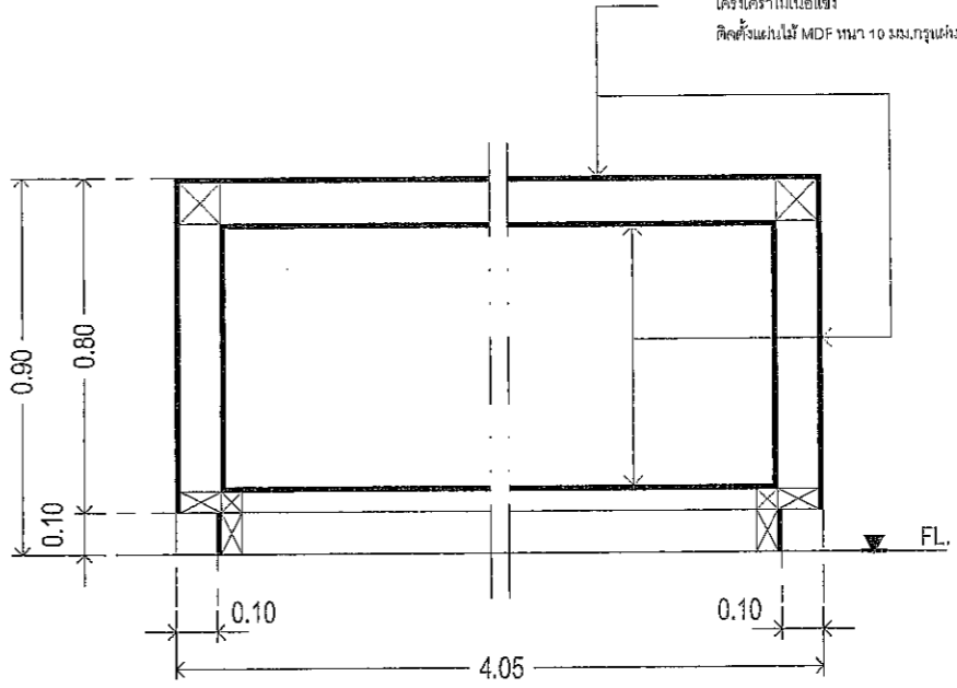
แบบขยายชุด RECEPTION COUNTER : รูปตัด B
