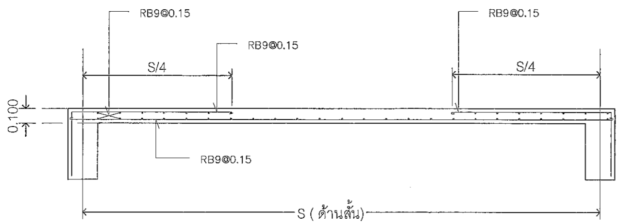
พื้น S3 SCALE 1:25 A3
