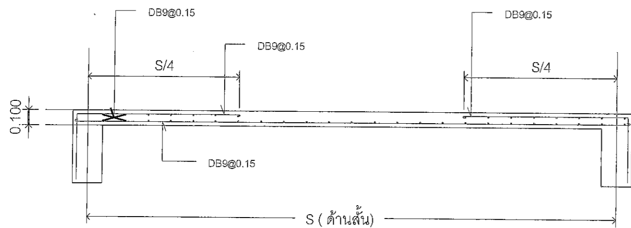
พื้น S3
