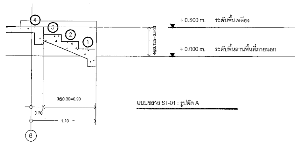
แบบขยาย ST-01, R-01 : ผังพื้น SC4 E 1.75 A3
