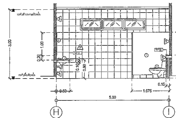
แบบขยายห้องน้ำ : รูปตัด B SCALE 1:100 A3
