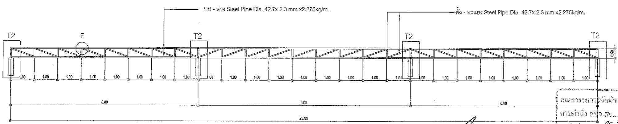
TRUSS T3A SCALE 1:100 A3
