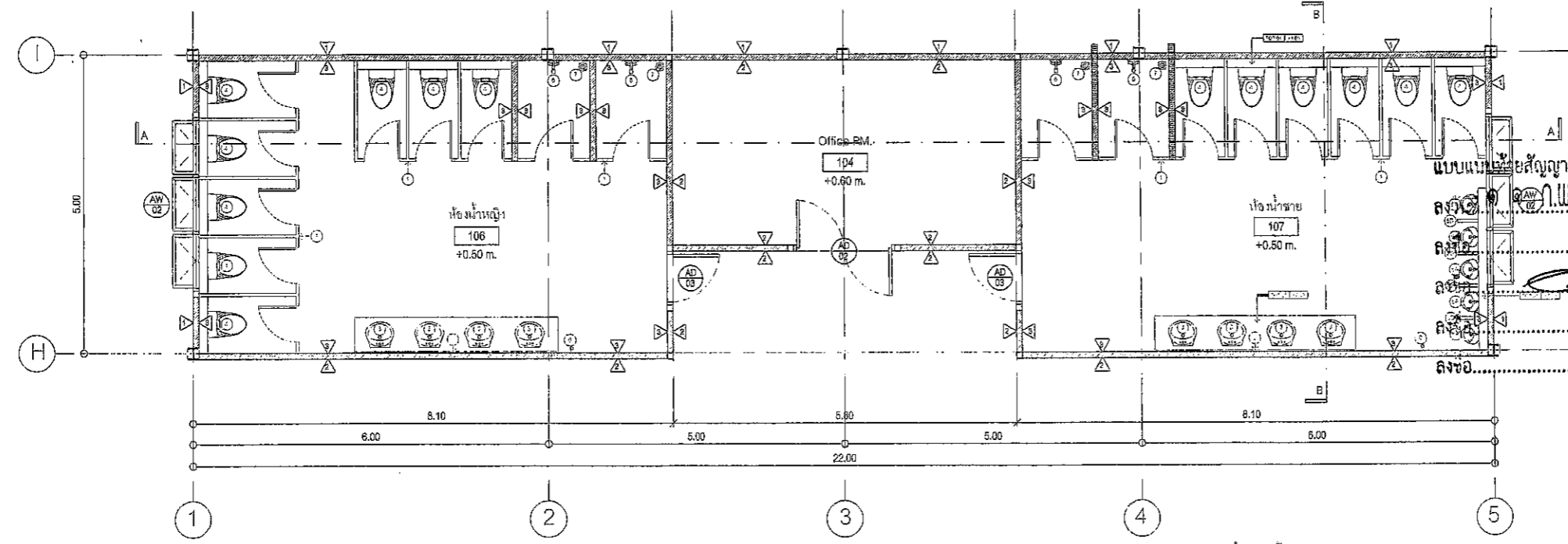
แบบขยายห้องน้ำ : สำพื้น SCALE 1:100 A3
