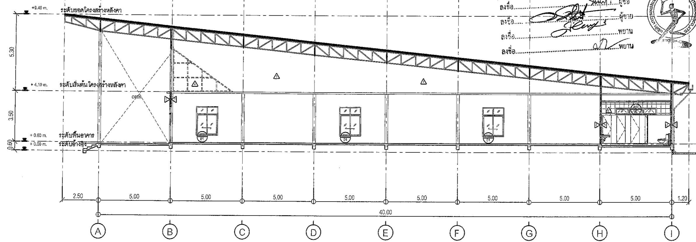
รูปตัด A SCALE 1:150 A3
