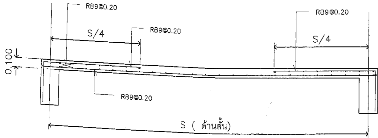
พื้น S1 SCALE 1:25 A3
