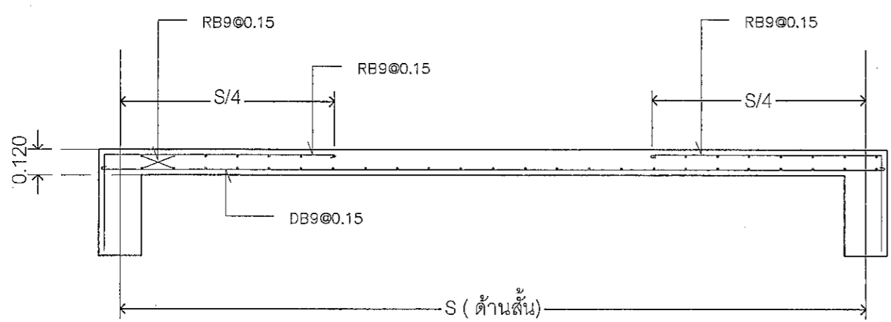
พื้น S2 SCALE 1:25 A3
