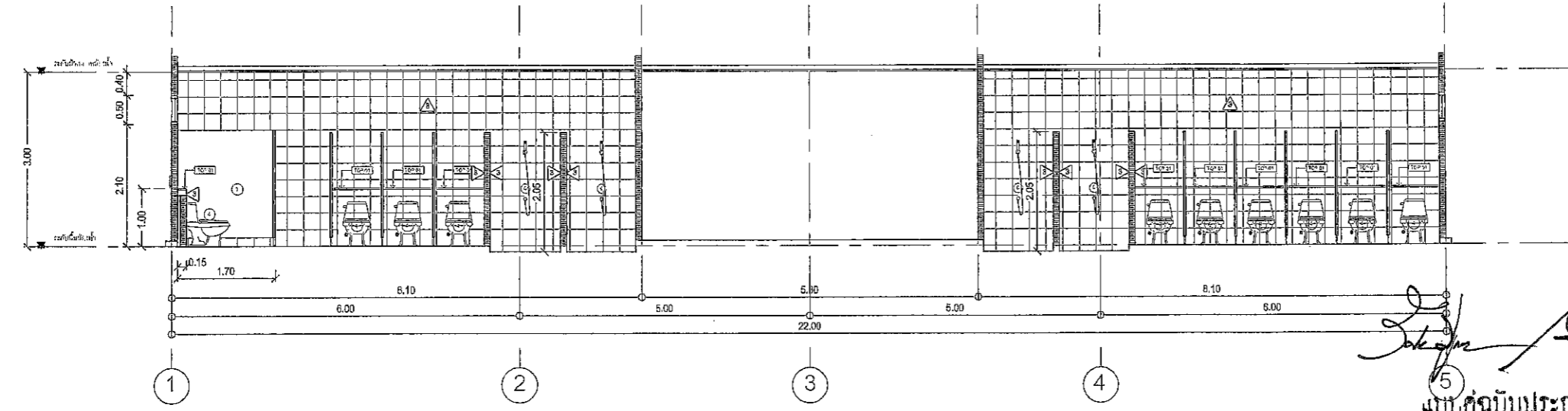
แบบขยายห้องน้ำ : รูปตัด A SCALE 1:100 A3
