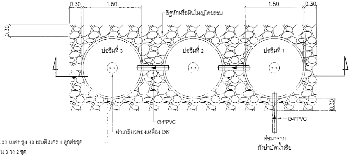
แปลนบ่อซีเมนต์
