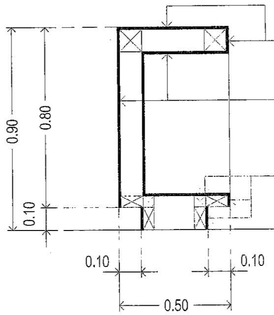
แบบขยายชุด RECEPTION COUNTER : รูปตัด A
