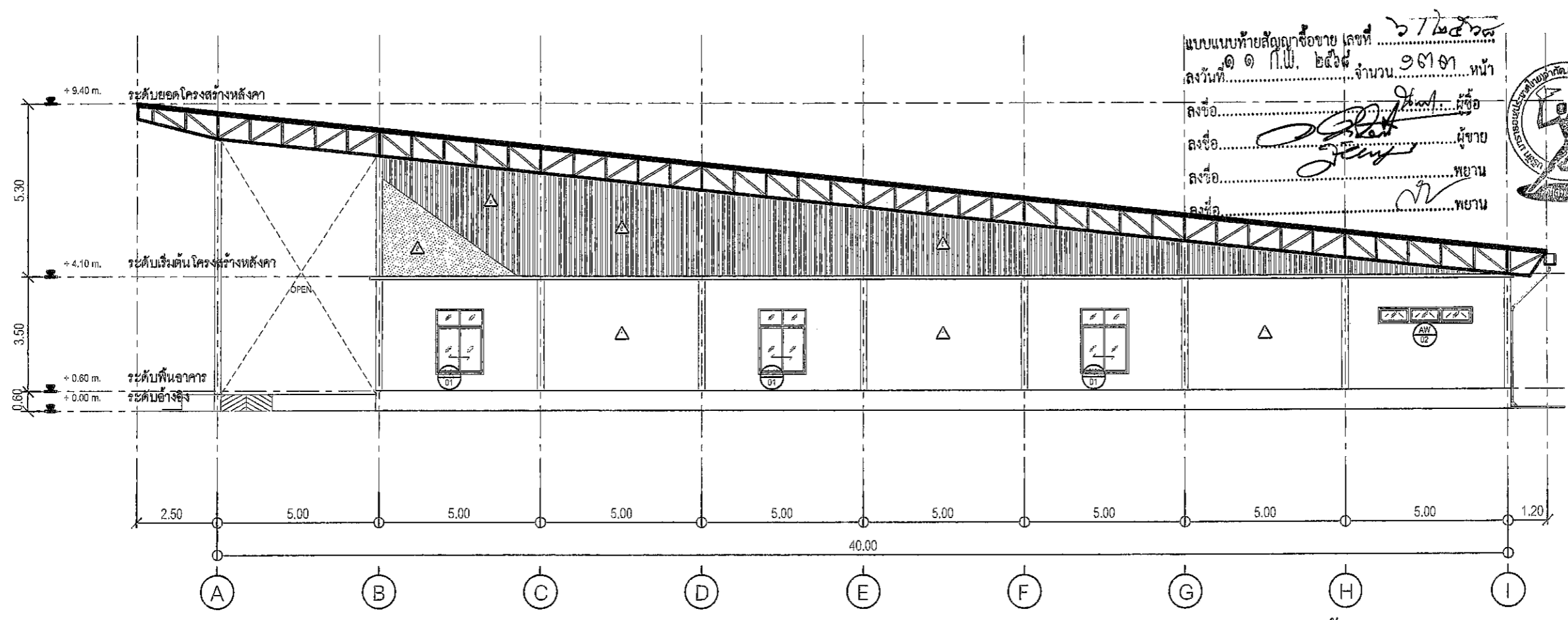
รูปด้าน 1 SCALE 1:150 A3
