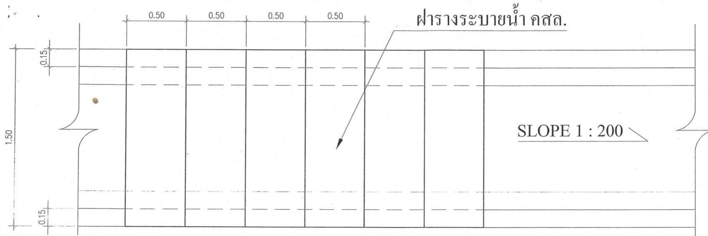
รูปแปลน รางระบายน้ำ
