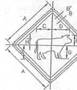
เว้นขอบป้าย สีเหลืองสะท้อนแสง เส้นขอบป้าย สีดำไม่สะท้อนแสง พื้นป้าย สีเหลืองสะท้อนแสง เครื่องหมาย สีดำไม่สะท้อนแสง
