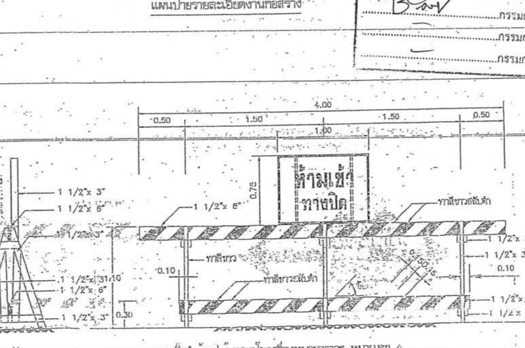
แผงกั้นที่ ดึงไม้ และป้ายเครื่องหมายจราจร หมายเลข ๔
