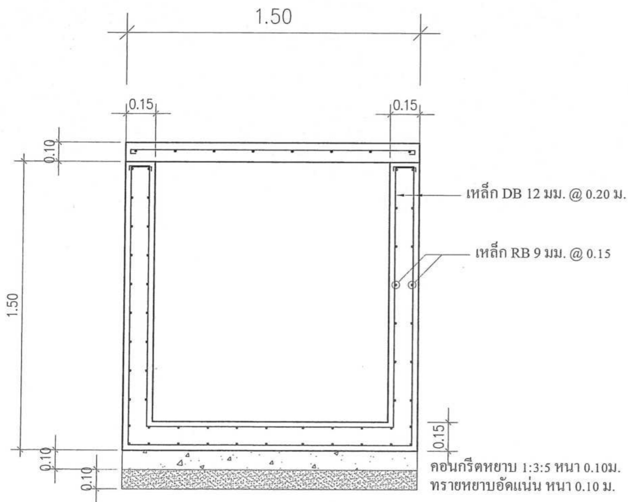
รูปตัดขยาย รางระบายน้ำ
