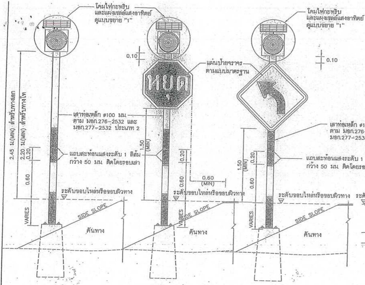
โคมไฟกะพริบ และแผงเซลล์แสงอาทิตย์ ดูแบบขยาย "1"
