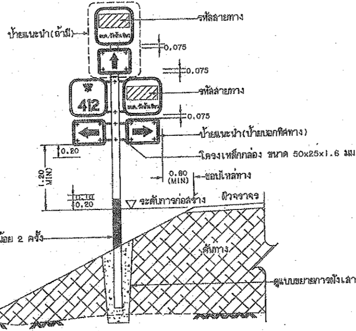
แสดงการติดตั้งเลาป้ายชุดระบุทิศทาง
