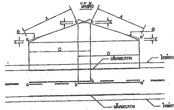
กรณีความกว้างสะพานมากกว่าความกว้างผิวจราจรบน
