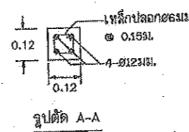
รูปตัดแสดงเสาป้าย
