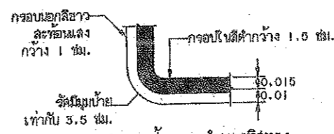
แสดงมุมป้ายแนะนำนอกทิศทาง (น-6 ถึง น-19)
