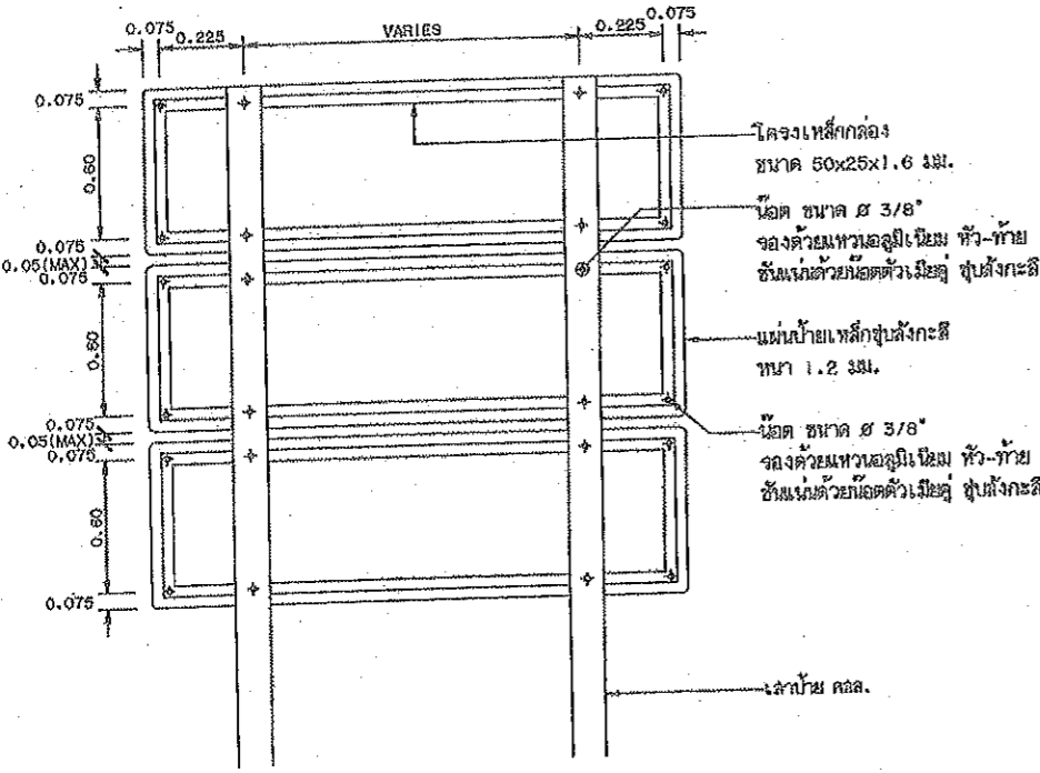
แสดงการยึดโครงเลาป้าย น-2 (ชุด) และ น-3 (ชุด)
