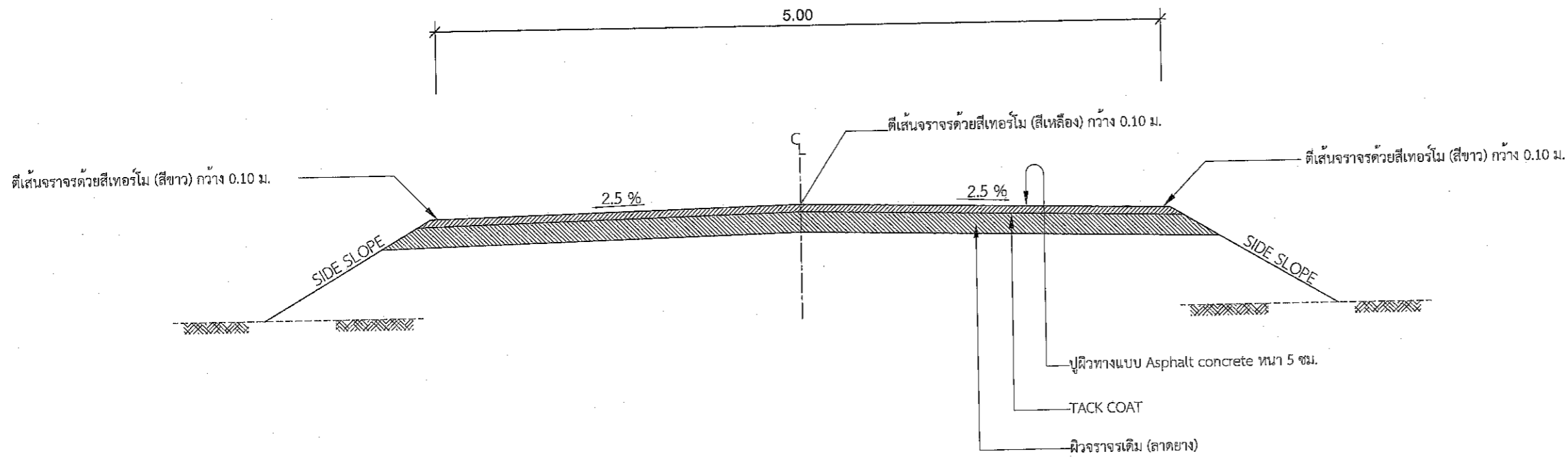
รูปตัดตามขวาง ASPHALT CONCRETE
