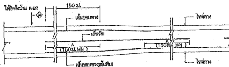
การขึ้นจากราคา กรณีความกว้างของบ่อจราจรลดลง
