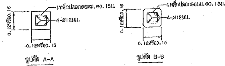
รูปตัดเลาป้าย (ดูหมายเหตุ ข้อ 4)
