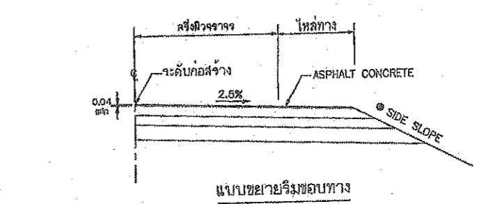
ถนนผิวจราจรแบบ ASPHALT CONCRETE ตารางแนะนำการออกแบบความหนาของชั้น โครงสร้างทาง (ระยะเวลาการออกแบบ 7 ปี)
