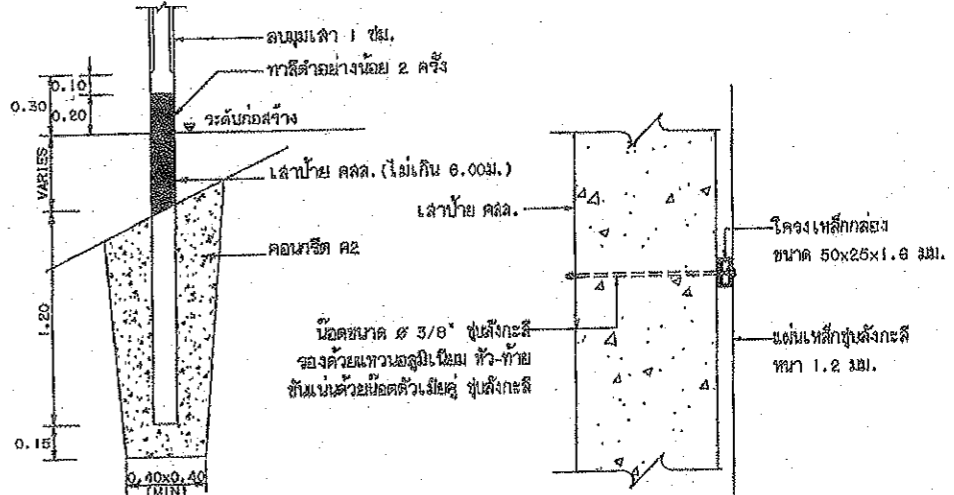
แสดงการฝังเลาป้าย
