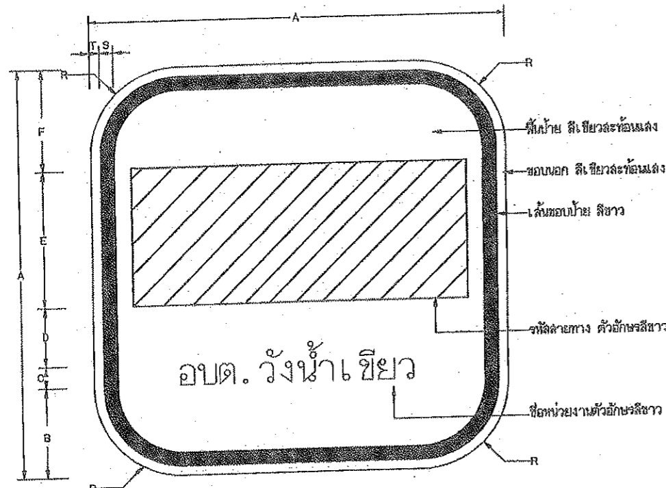
แสดงมุมป้ายแนะนำ (น-1)
