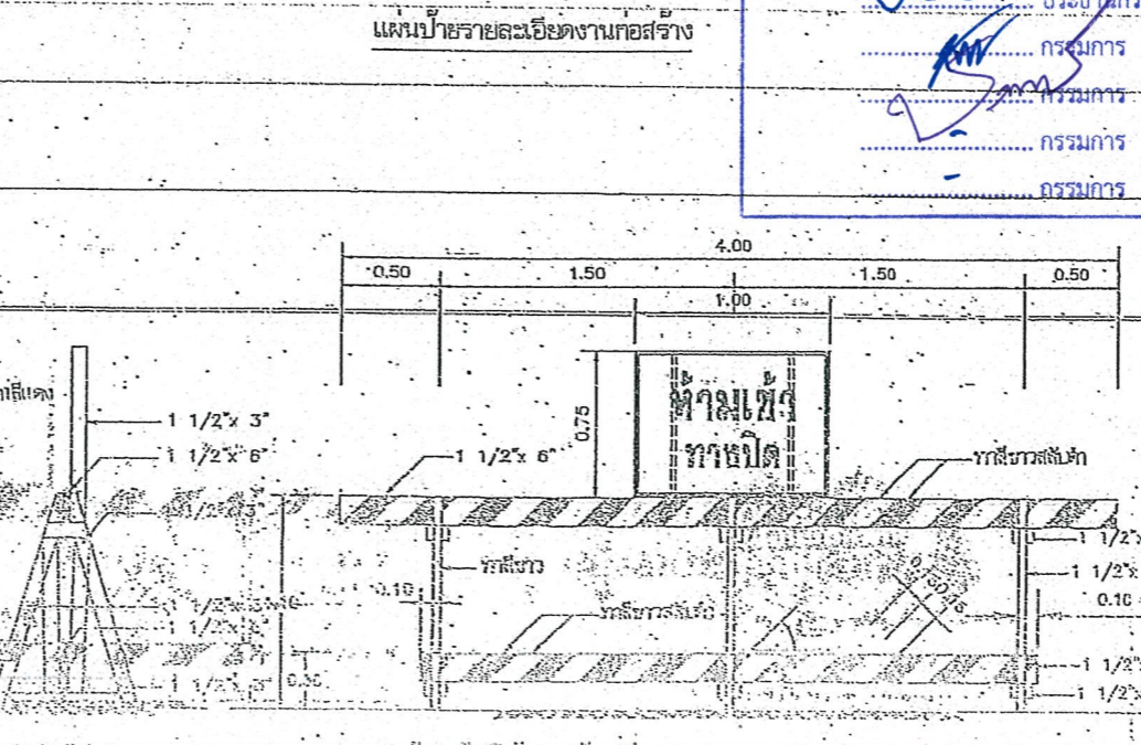
แปลนพื้นที่ด้วยไม้ และป้ายเครื่องหมายจราจร หมายเลข 4
