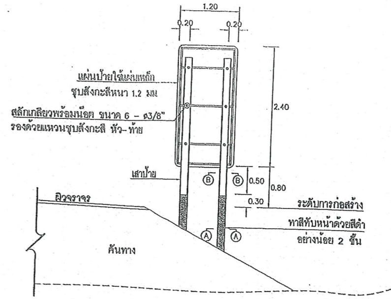
แสดงการติดตั้งป้าย (ด้านหลัง) ไม่แสดงมาตราส่วน
