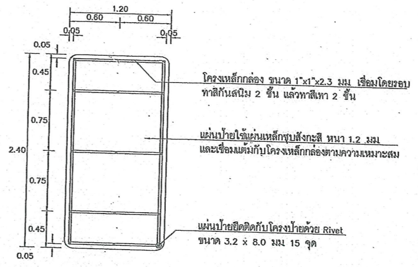
แสดงการยึดแผ่นป้ายกับโครงเหล็ก ไม่แสดงมาตราส่วน
