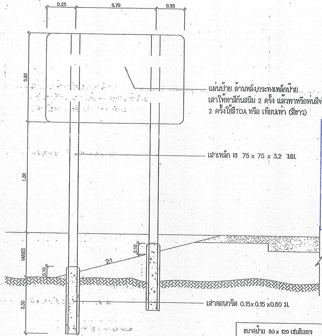
แสดงการปักเสาสัญ
