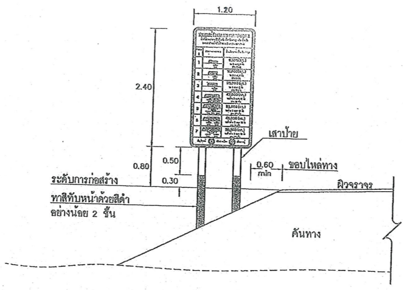
แสดงการติดตั้งป้าย (ด้านหน้า) ไม่แสดงมาตราส่วน
