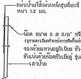
รายละเอียดด้านหลังป้าย น-5
