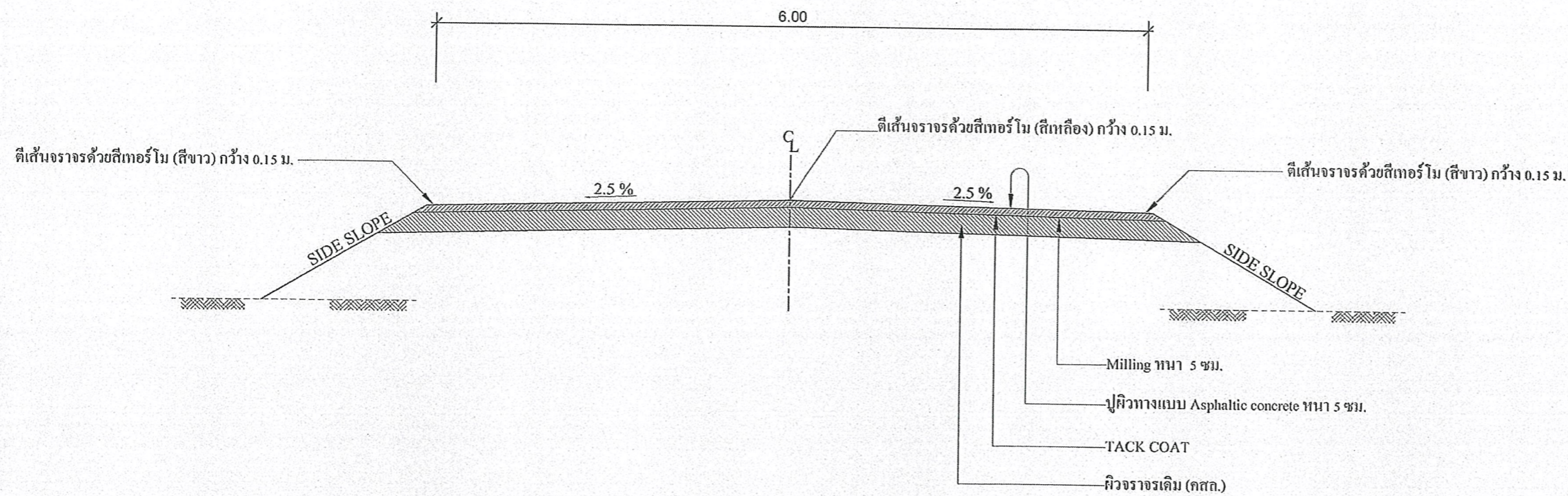
รูปตัดตามขวาง ASPHAL CONCRETE
