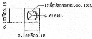
รูปตัดเสาป้าย
