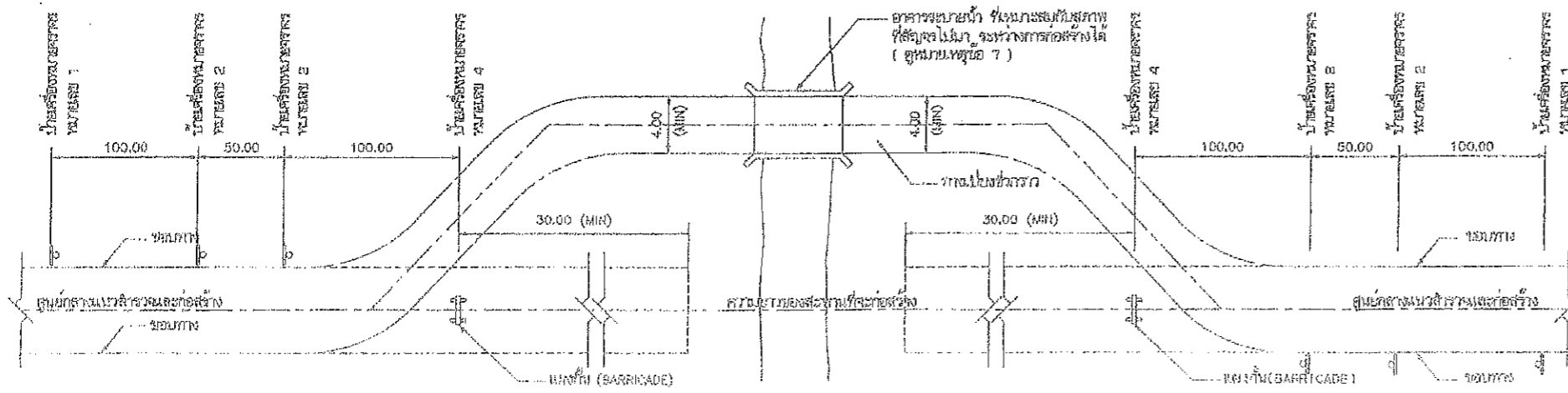
แปลนติดตั้งแท่งของทางเบี่ยง และด้านหน้าของสิ่งกีดขวางจราจร
