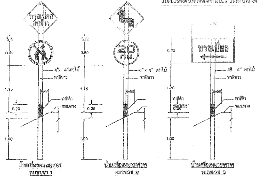
แปลนติดตั้งแท่งของทางเบี่ยง และด้านหน้าของสิ่งกีดขวางจราจร
